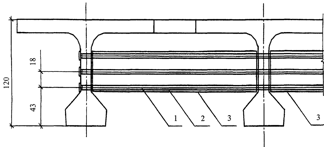
Рис. 3.6. Расположение канатов в пролетном строении длиной 21 м по типовому проекту инв. № 384/27:
