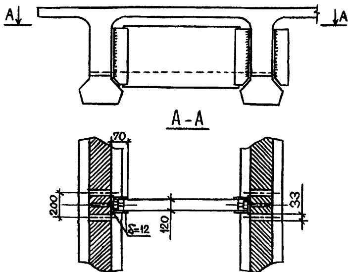
Рис. 3.8. Направляющие элементы для вставных диафрагм.
