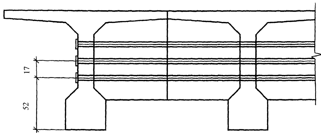
Рис. 3.4. Расположение канатов в трех уровнях для предварительно напряженной балки длиной 22,16 м с диафрагмами. Размеры даны в сантиметрах
