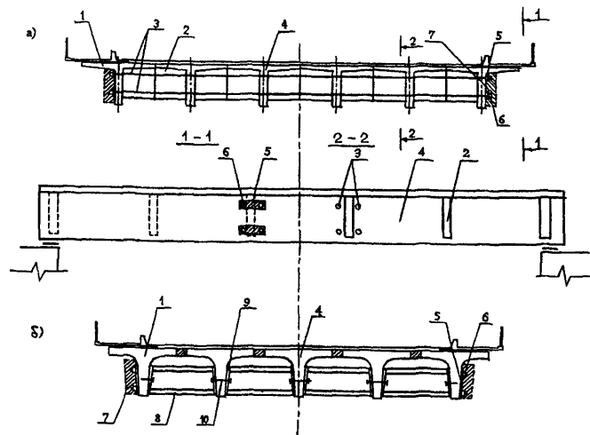
Рис. 3.1. Схема расположения канатов класса К-7 в диафрагменном (а) и в бездиафрагменном (б) пролетном строении: 1 - крайняя балка; 2 - диафрагма; 3 - канаты класса К-7; 4 - средняя балка; 5 - фасадная опорная плита; 6 - анкер; 7 - бетон омоноличивания; 8 - вставная диафрагма; 9 - направляющие к вставным диафрагмам; 10 - болты для крепления вставных диафрагм
