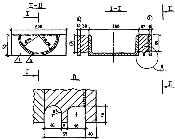
Рис. 4. Отгибальное устройство для усиления каркасных балок двумя пучками из 12 шт. высокопрочных проволок диаметром 5 мм класса В (а) и четырьмя пучками из одиночных арматурных канатов класса К-7 (б): 1 - швеллер; 2 - отгибальный элемент. Размеры даны в миллиметрах.
