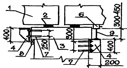
Рис. 5.5. Установка домкратов на инвентарные (а) и отдельные (б) столики, закрепляемые на промежуточной опоре:
