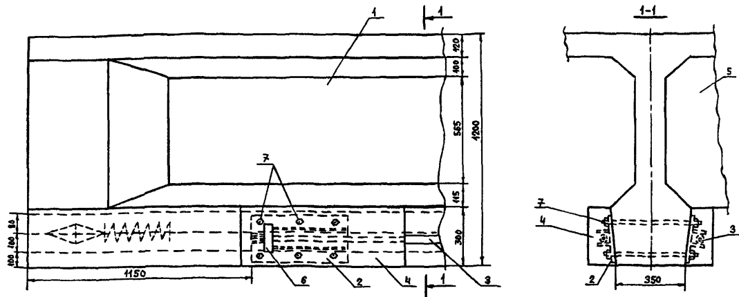
Рис. 3. Схема усиления предварительно напряженных балок мощными пучками: 1 - усиливаемая балка; 2 - накладной упор; 3 - пучок из арматурных канатов класса К-7 или высокопрочных проволок; 4 - бетон омоноличивания упора; 5 - диафрагма балки; 6 - анкер; 7 - болты для крепления упора. Размеры даны в миллиметрах.
