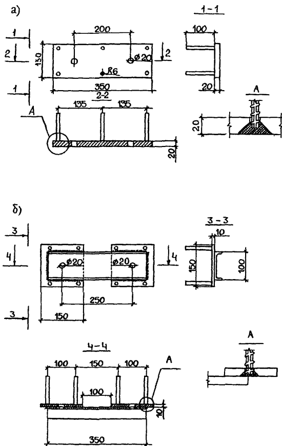
Рис. 3.7. Конструкция плоских (а) и с ребрами (б) опорных плит. Размеры даны в миллиметрах.
