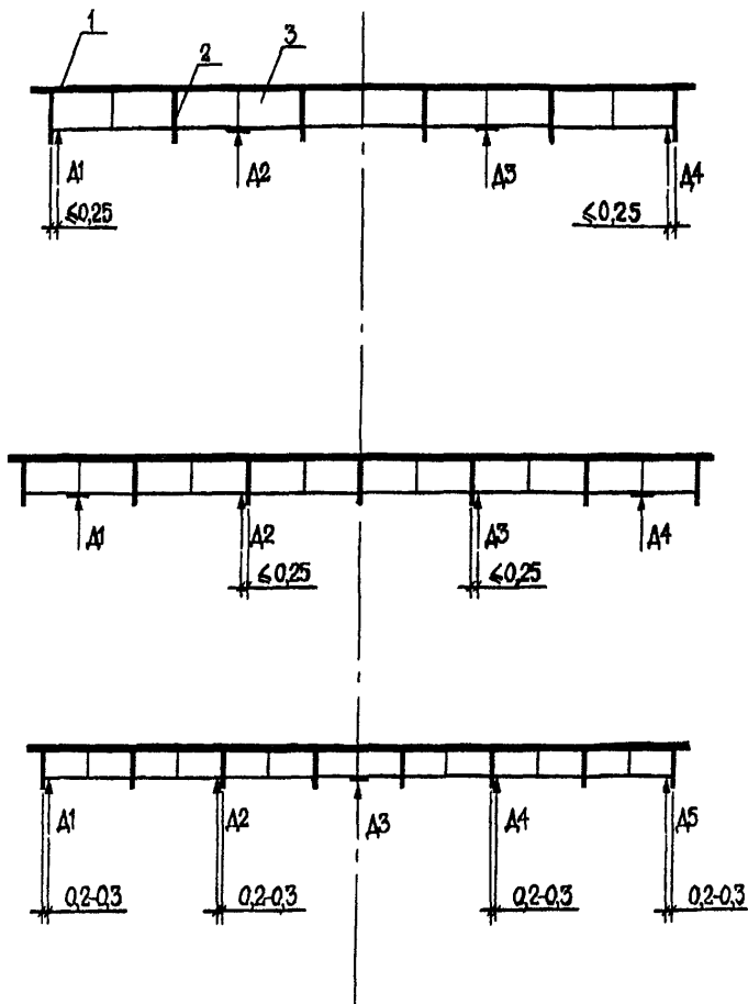
Рис. 5.2. Расположение домкратов в диафрагменных пролетных строениях:
