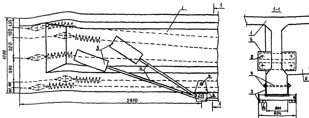
Рис. 2. Схема усиления балок с напрягаемой арматурой:
