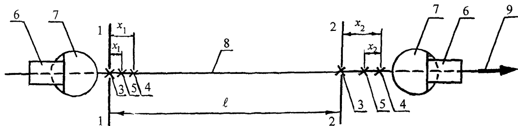
Рис. Схема измерения вытяжки напрягаемой арматуры:
