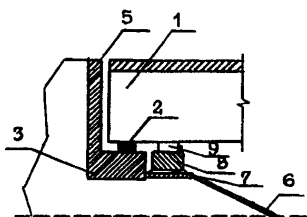
Рис. 5.4. Расположение домкратов на устое в бездиафрагменном пролетном строении с устройством ниши (а) и с использованием свай (б):
