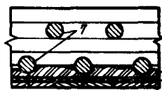
Рис.5. Устройство дренажа в конструкциях из буронабивных свай: 1-окно; 2-дренажная труба; 3-геотекстиль; 4-плиты; 5-грунт; 6-ростверк; 7-буронабивные сваи
