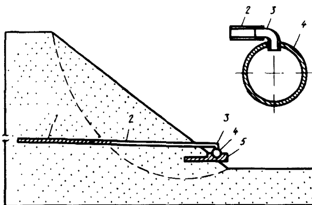
Рис.9. Сброс грунтовых вод по коллектору: 1-водоприемная часть дрены; 2-водоотводная часть дрены; 3-переходник; 4-коллектор; 5-опора
