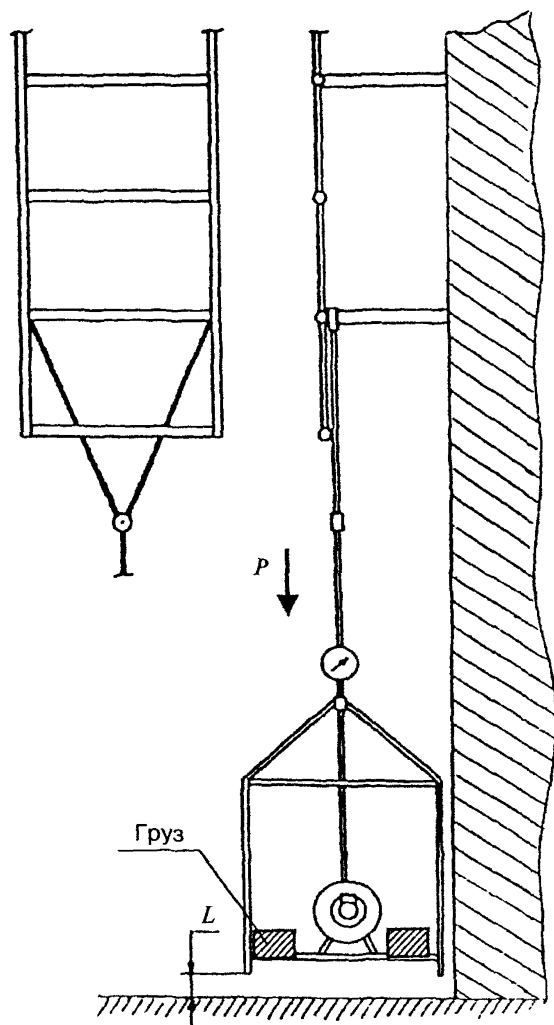
Рисунок 2. Испытание на прочность балки крепления вертикальной лестницы (высота отрыва площадки от земли L = 100\text{—}200\text{ мм} )
