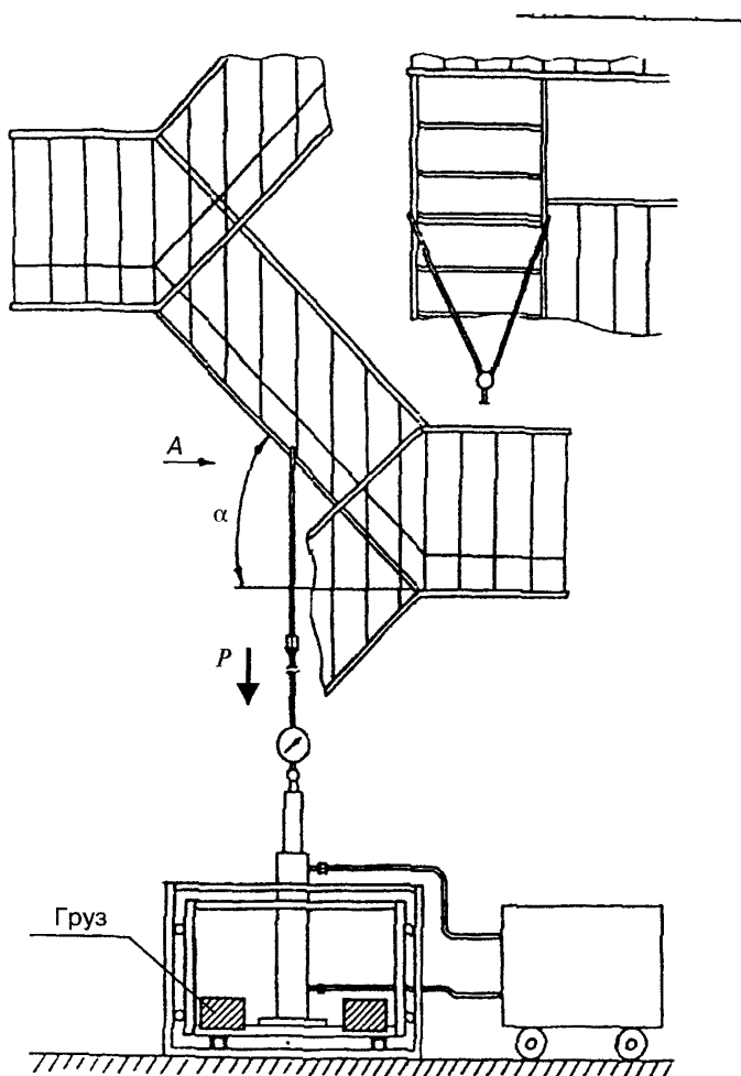
Рисунок 3. Испытание на прочность марша лестницы
