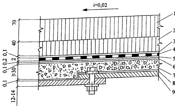
Рис. 2. Одежда ездового полотна по стальной ортотропной плите с соединениями на высокопрочных болтах: 1 – рабочий слой асфальтобетонного покрытия; 2 – защитный слой асфальтобетона; 3 – мастика «Полибит»; 4 – рулон «Поликров-Р200»; 5 – мастика «Полибит-М140»; 6 – мастика «Полибит»; 7 – выравнивающий слой из литого или плотного мелкозернистого асфальтобетона; 8 – грунтовка; 9 – настильный лист ортотропной плиты Примечание. Если поверхность ортотропной плиты не загрунтована на заводе, позиция «8» отсутствует.
