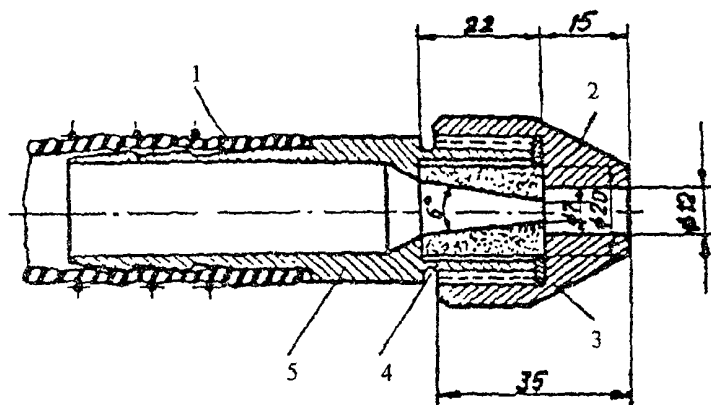
Рис. Б.2. Минералокерамическое сопло: 1 - шланг; 2 - накидная гайка; 3 - уплотняющая прокладка; 4 - рабочая часть; 5 - соплодержатель
