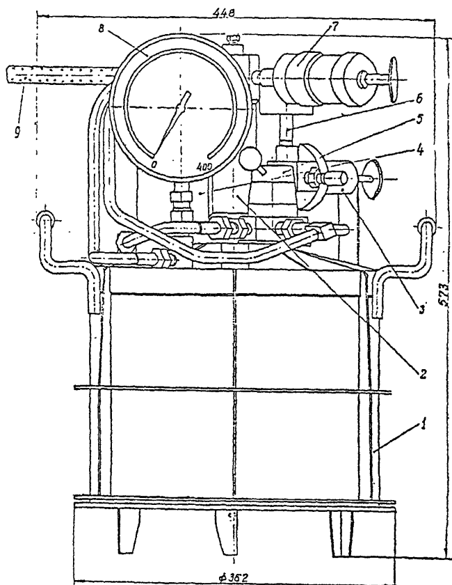
Рис. И.5. Пневмогидравлический насос НГП-250: 1 - пневмоцилиндр; 2 - гидроцилиндр; 3 - воздушный редуктор; 4 - распылитель; 5 - пневмораспределитель; 6 - трубка; 7 - отсекатель; 8 - манометр; 9 - шланг
