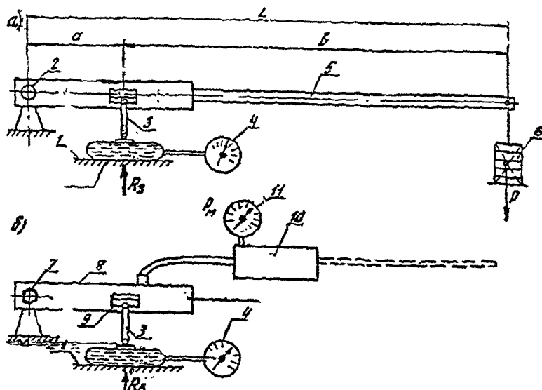
Рис. К.2. Принципиальная кинематическая и гидравлическая схемы тарирования гидравлических ключей:
