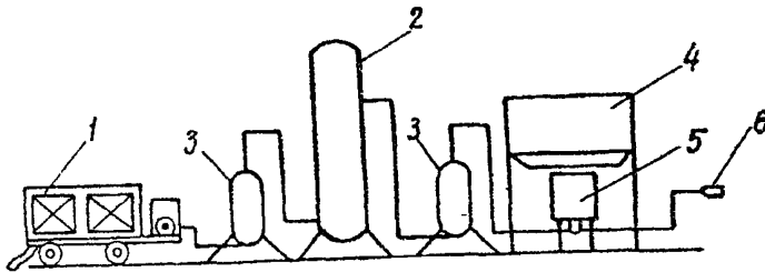
Рис. 1. Схема пескоструйной установки.
