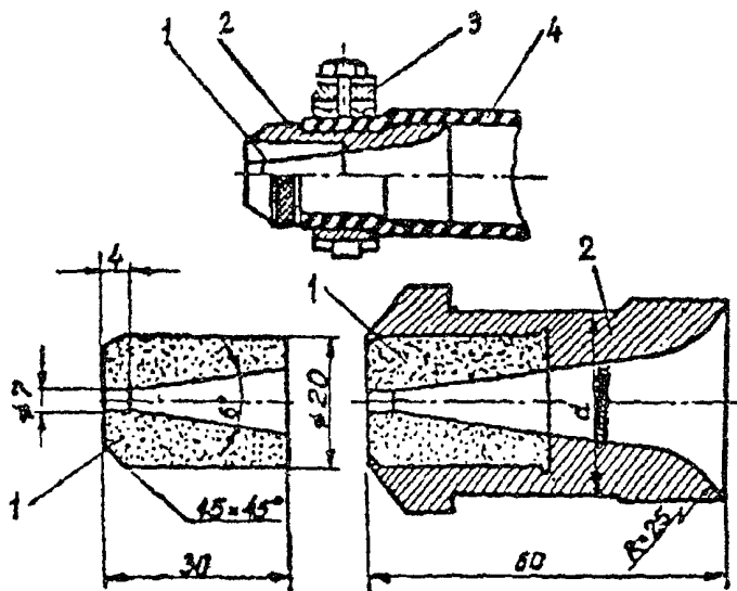
Рис. Б.3. Металломинералокерамическое сопло: 1 - минералокерамическая вставка; 2 - соплодержатель; 3 - хомуттик; 4 - шланг; d - диаметр шланга
