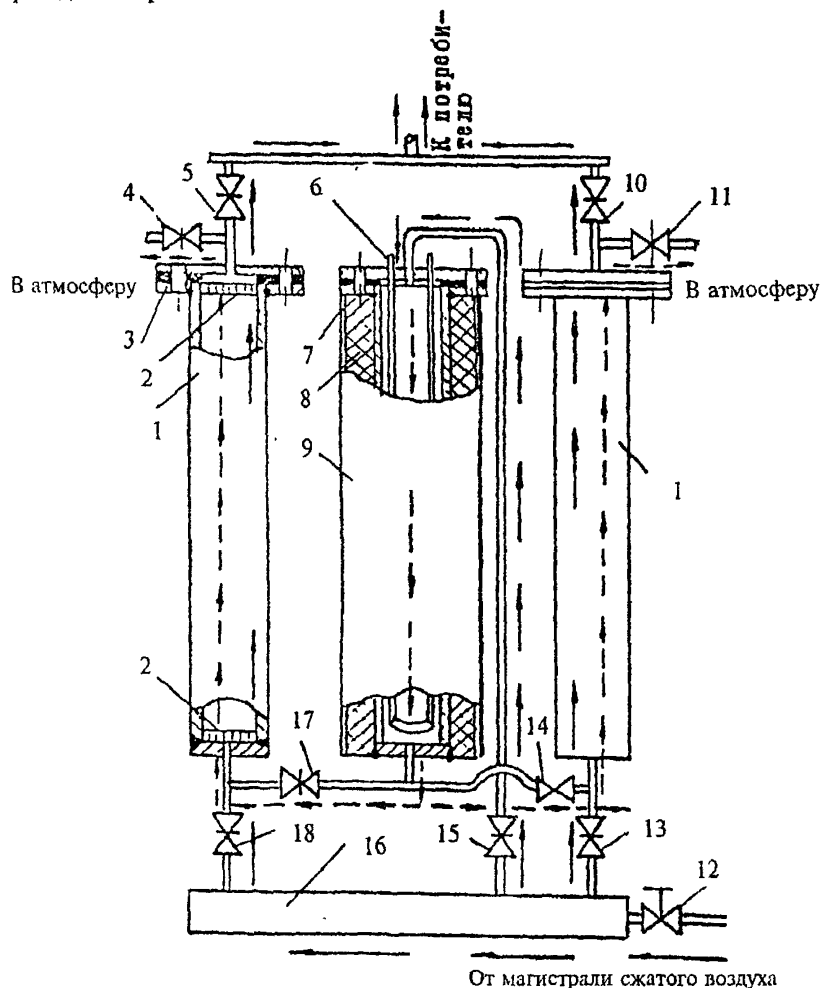
Рис. В.2. Схема переносного масляного очистителя:
