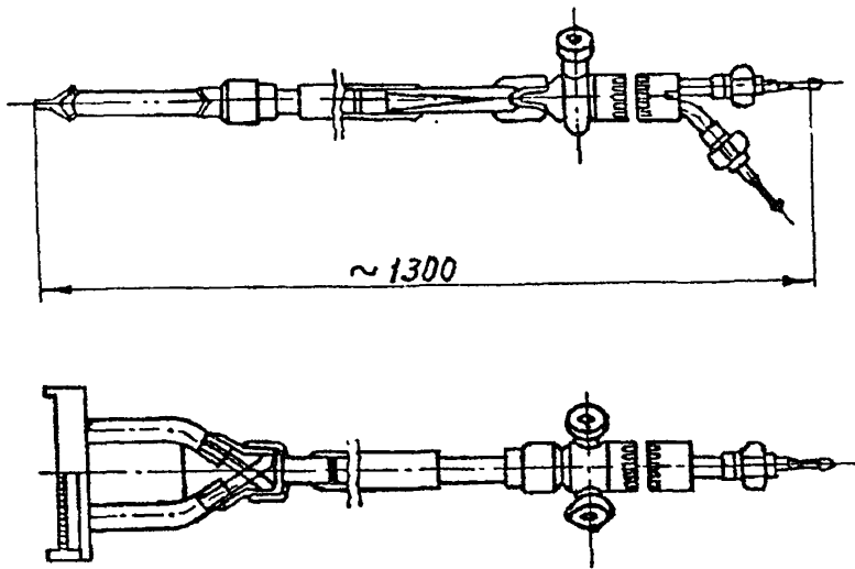
Рис 4. Широкопламенная кислородно-ацетиленовая горелка ГАО-60
