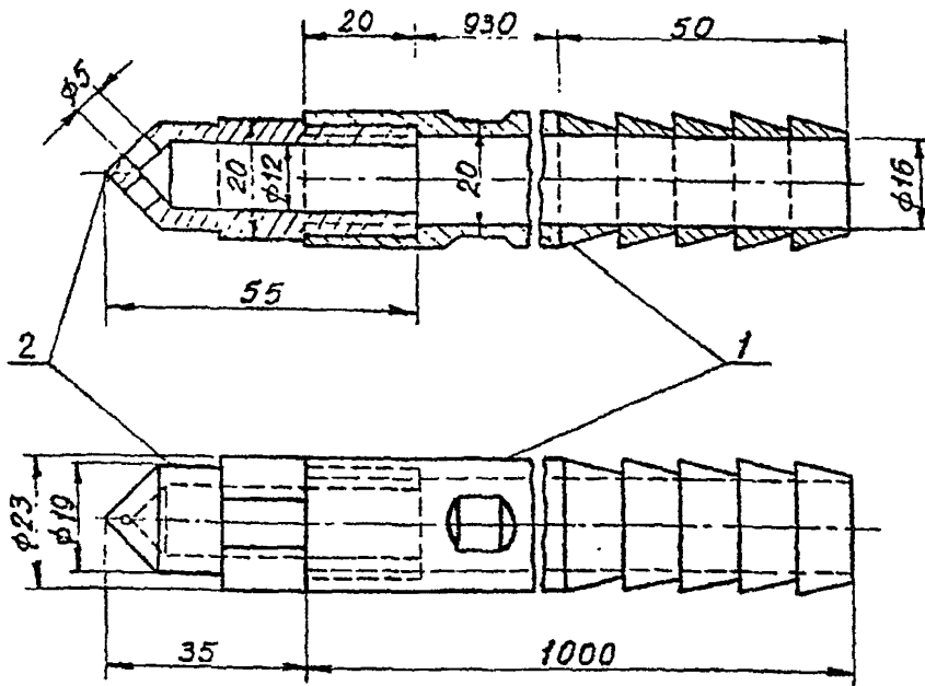
Рис. Б.4. Сопло для очистки поверхностей в "вилках": 1 - соплодержатель; 2 - рабочая часть
