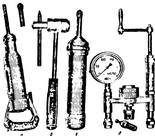
Рис.4. Приборы механического действа: а - типа КМ со стержневым ударником; б - ударник с шариковым наконечником для прибора КМ; в - эталонный молоток; г - типа ХСП; д - типа ГПНВ-5.
