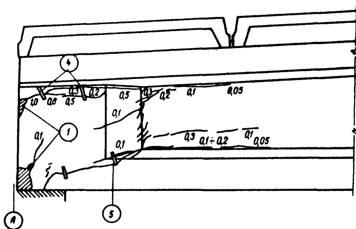
Рис 3 Схема зарисовки трещин на опорном участке балки 16В-18-3 серии ПК-01-06 1-сколы бетона, 2-стержни \phi 6 мм, 3-деформированные прутья; 4-выпуклый наплыв, 5-разрыв напла по трещине; 6-участок балки недоступный для осмотра. Цифры у трещин обозначают величину их раскрытия в мм.
