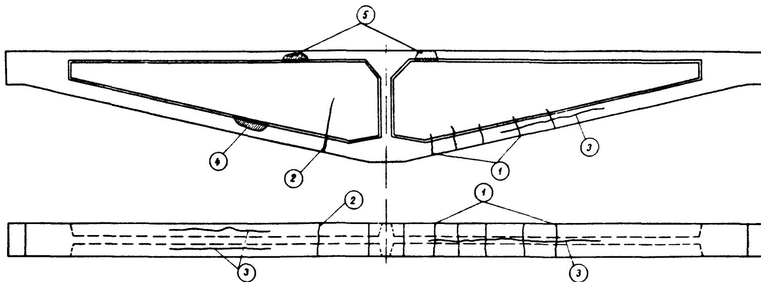
Рис. 13 Характерные дефекты в натянутой балке.
