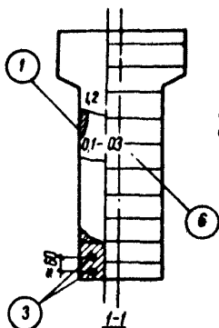
Рис 3 Схема зарисовки трещин на опорном участке балки 16В-18-3 серии ПК-01-06 1-сколы бетона, 2-стержни \phi 6 мм, 3-деформированные прутья; 4-выпуклый наплыв, 5-разрыв напла по трещине; 6-участок балки недоступный для осмотра. Цифры у трещин обозначают величину их раскрытия в мм.
