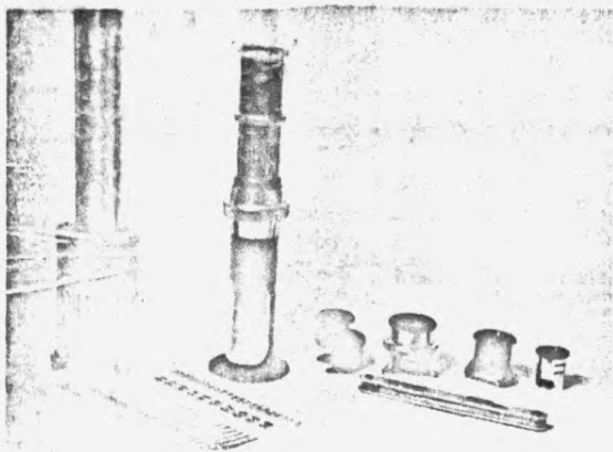
Рис. 1. Инструменты для определения величины раскрытия трещин 1 - трубка Бринелля, 2 - отсчетный микроскоп МПБ-2 - \times 24 , 3 - градуированные лупы Польди - \times 12 , 4 - градуированная лупа Польди - \times 16 , 5 - визирная лупа - \times 10 , 6 - графарет на прозрачной пленке, 7 - шуп.
