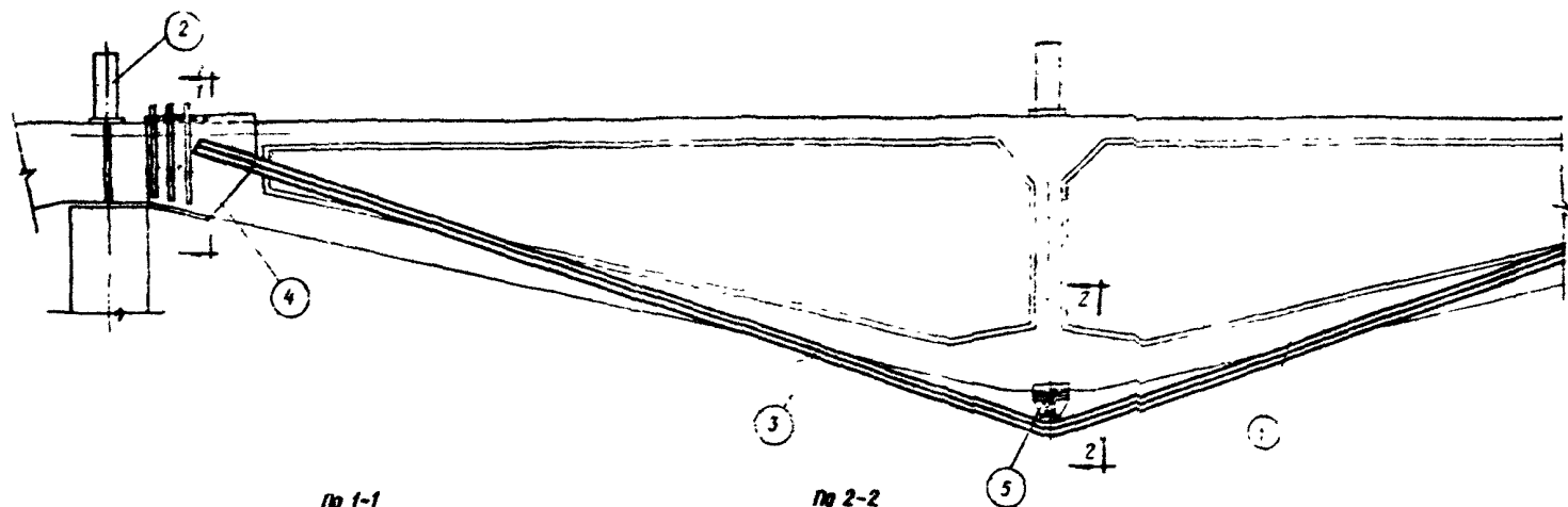
по 1-1
