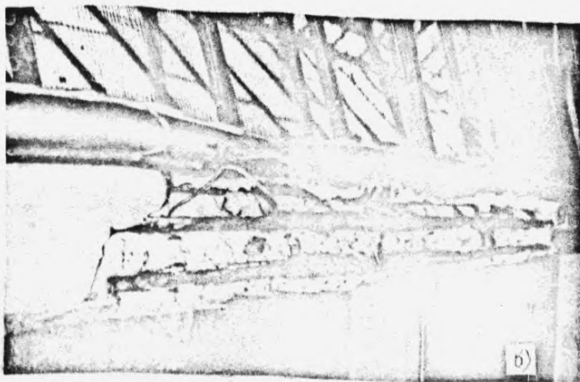
Рис.7. Разрушение железобетонных балок перекрытия в результате коррозии арматуры
