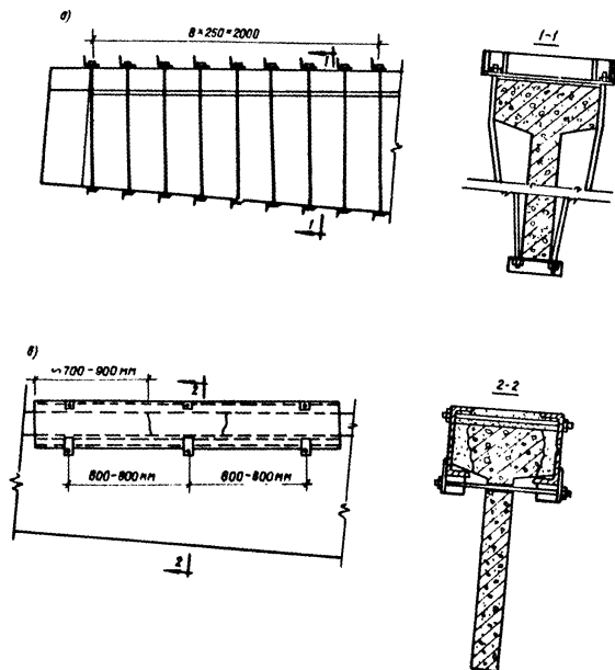
Рис.12. Способы усиления балки: а) усиление опорного участка наружными натяжными хомутами, б) усиление обоймой поврежденного участка полки.
