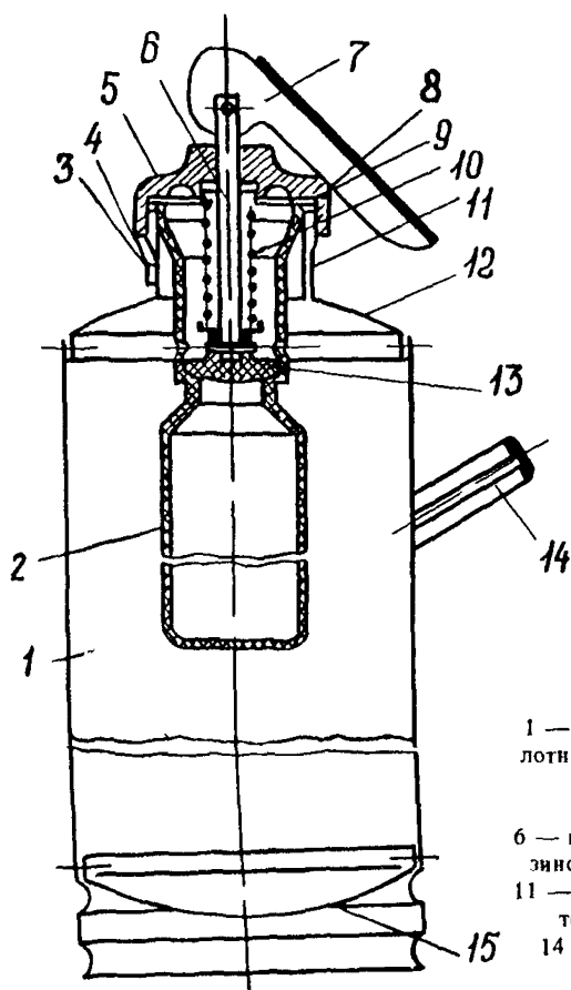
Рис. 1. Огнетушитель ОХП-10:
