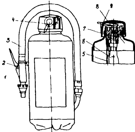
Рис. 12. Общий вид ручного порошкового огнетушителя ОП-5:
