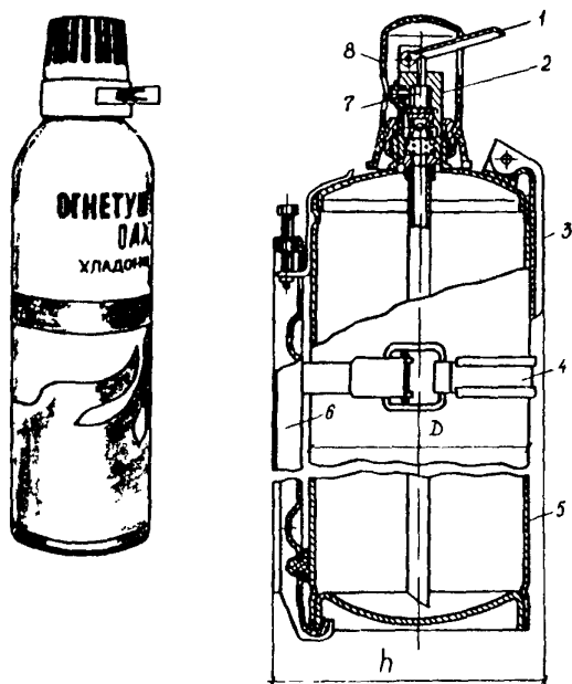
Рис. 11. Хладоновый огнетушитель ОУБ-3А (ОУБ-7А):
