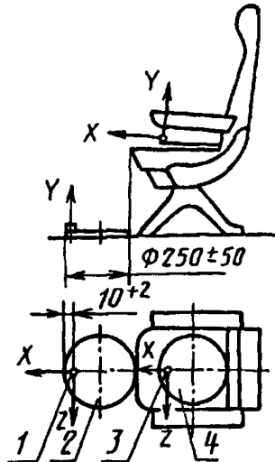
1, 3 — точки измерения; 2, 4 — лист Черт. 3
