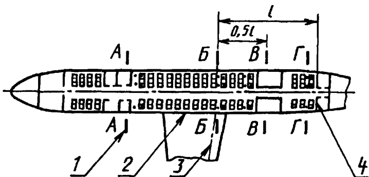
A, B, B, \Gamma — сечения; l — плоскость вращения внутренних винтов; 2 — корневая нервюра; 3 — задний лонжерон; 4 — задняя стенка пассажирской кабины Черт. 5
