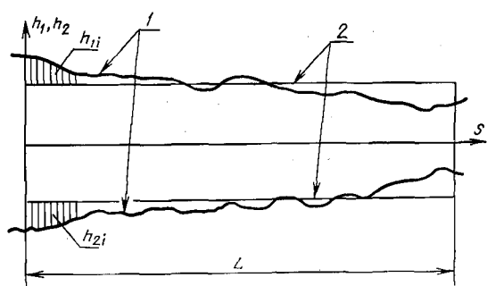
1 — реальный профиль; 2 — средний профиль продольного сечения
