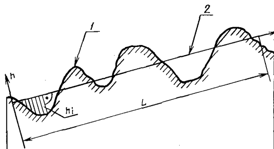
1 — реальный профиль; 2 — средняя прямая
