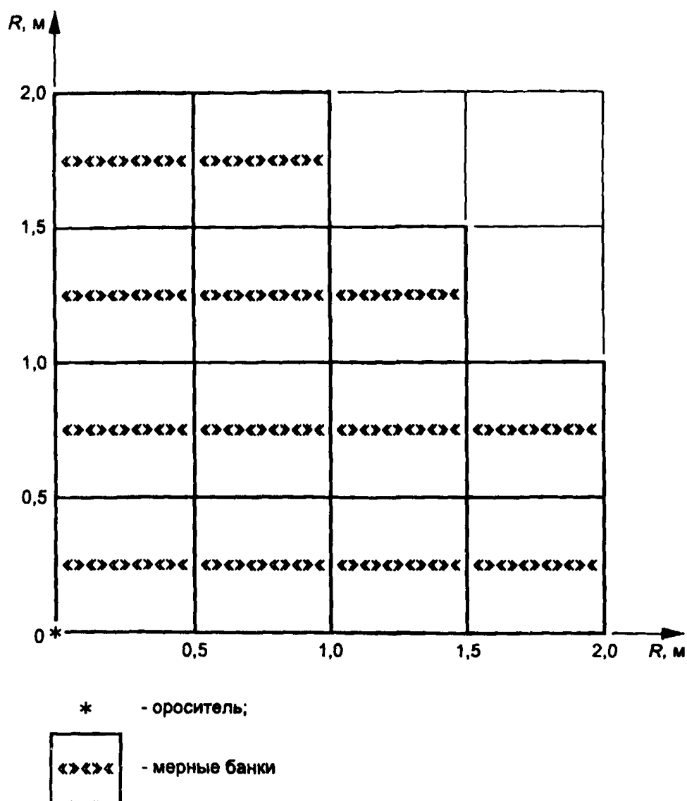
Рисунок 7 — Схема расположения мерных банок при испытаниях пенных оросителей
