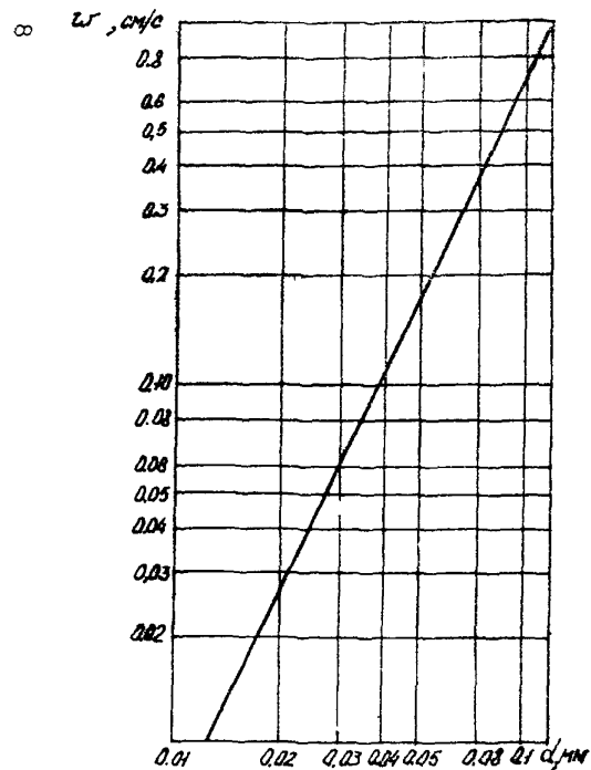
Рис.3. График для определения гидравлической крупности частиц песка
