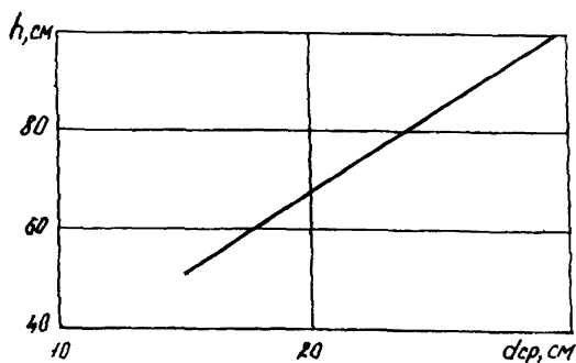
Рис. IП. Зависимость глубины шурфа от среднего размера наиболее крупных частиц
