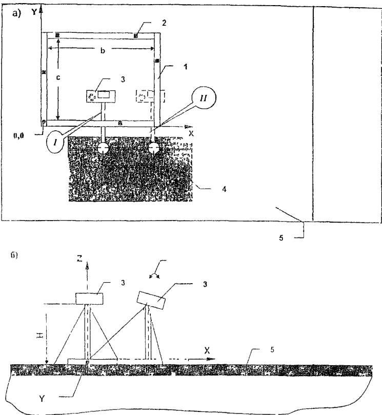
Рис. II-7.1. Схема элементов фотосъемки:
