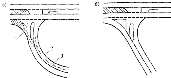
Рис. 8.7. Зрительное перекрытие островками неправильного направления движения:
