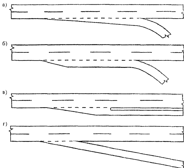
Рис. 9.2. Типы переходно-скоростных полос
