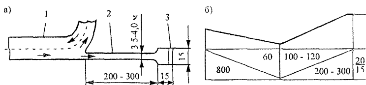
Рис. 5.1. Схема аварийного съезда:
