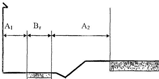
Рис. 11.1. Тротуар в населенном пункте:
