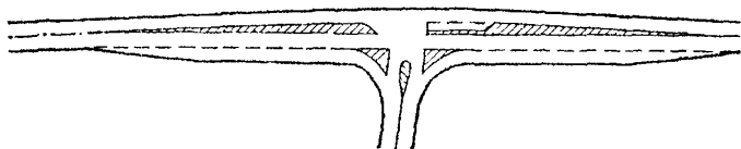
Рис. 8.8. Направляющие островки на примыкании в одном уровне
