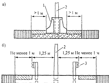
Рис. 15.1. Схема заделки в грунт опор освещения: а – при благоприятных условиях; б – в пучинистых грунтах; в – при наличии подземных коммуникаций; 1 – опора; 2 – оголовок; 3 – свая; 4 – деревянный короб; 5 – бетонный фундамент; 6 – металлический Г-образный фундамент
