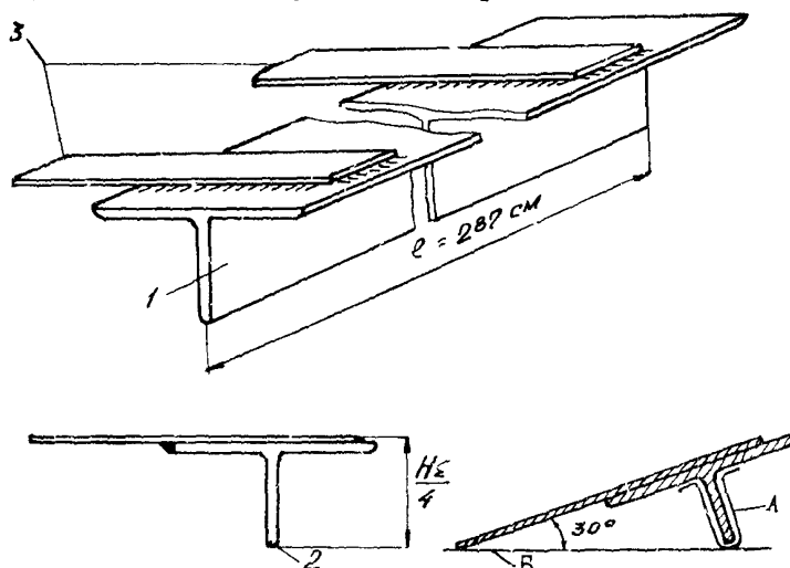
Шаблон для устройства швов в свежесуложенном бетоне А-пленка; Б-поверхность бетона
