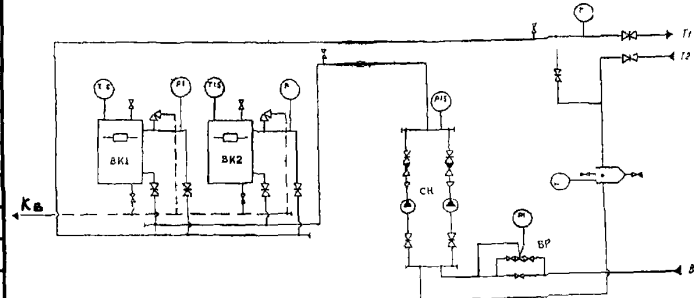
Принципиальная тепловая схема электрокотельной с двумя электродными котлами для закрытой системы отопления
