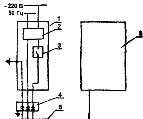
СХЕМА ПОДКЛЮЧЕНИЯ
