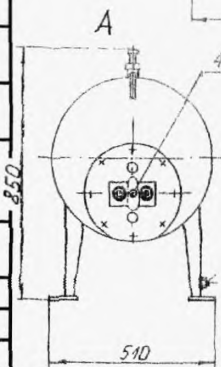
Рис.1. Общий вид электронагревателя типа САО - И1
