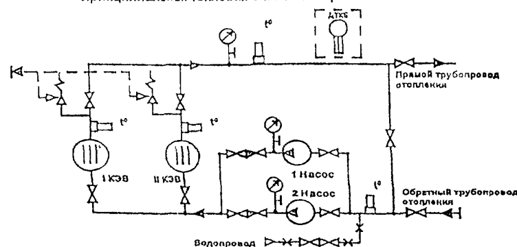
Принципиальная тепловая схема электрокотельной отопления.
