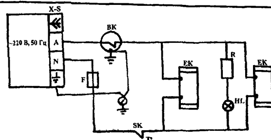
СХЕМА ЭЛЕКТРИЧЕСКАЯ ПРИНЦИПИАЛЬНАЯ
