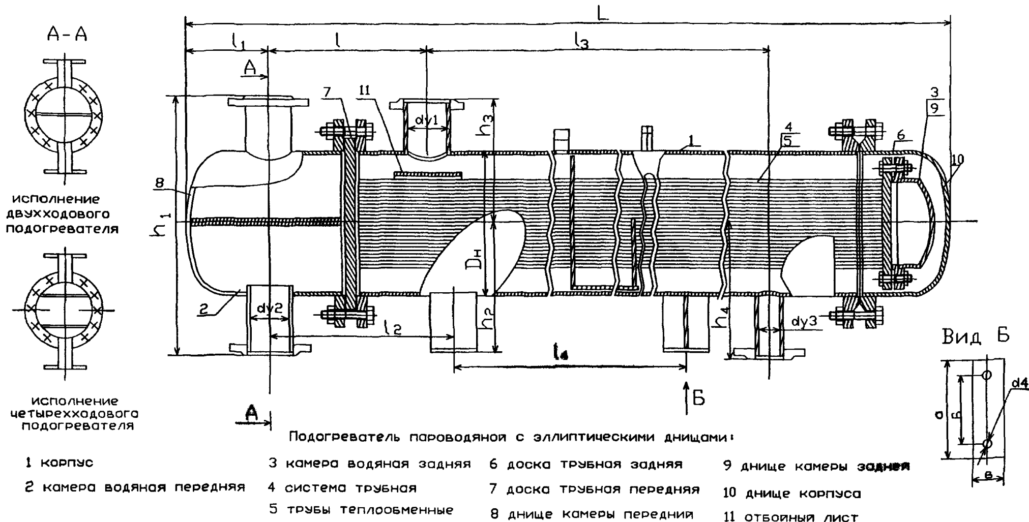
Габаритные и присоединительные размеры
