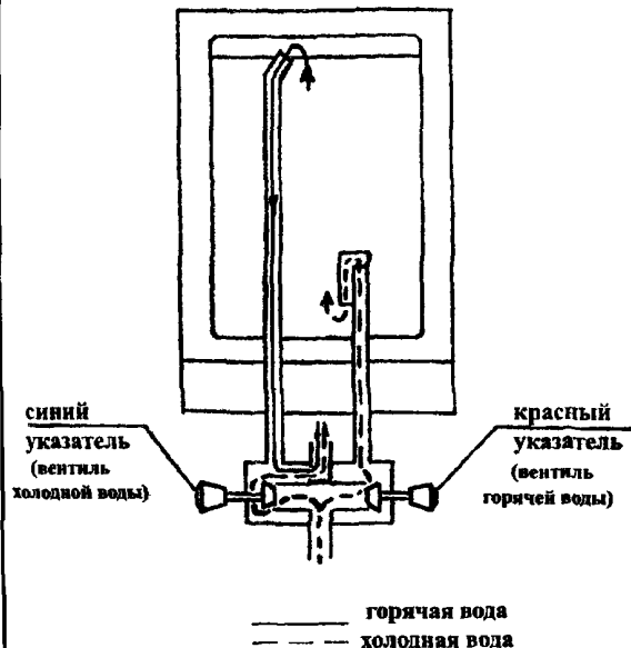
СХЕМА РАБОТЫ ЭЛЕКТРОВОДОНАГРЕВАТЕЛЯ
