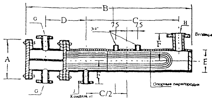
Блок пароводяного подогревателя типа ППРУ с охладителем конденсата типа ПВРУ
