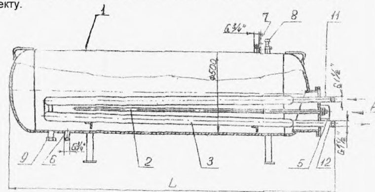
Рис.1. Общий вид электронагревателя типа САО - И1
