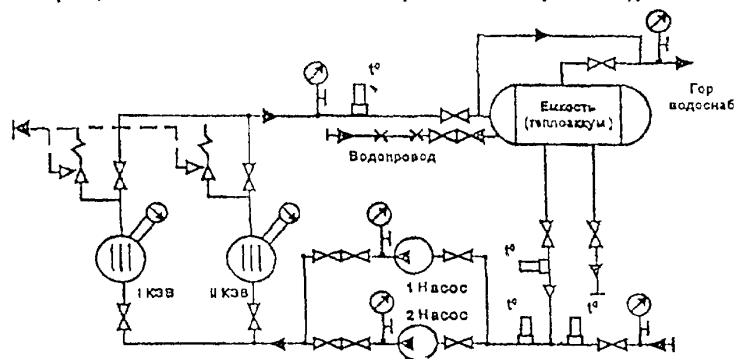
Принципиальная тепловая схема электрокотельной горячего водоснабжения.
