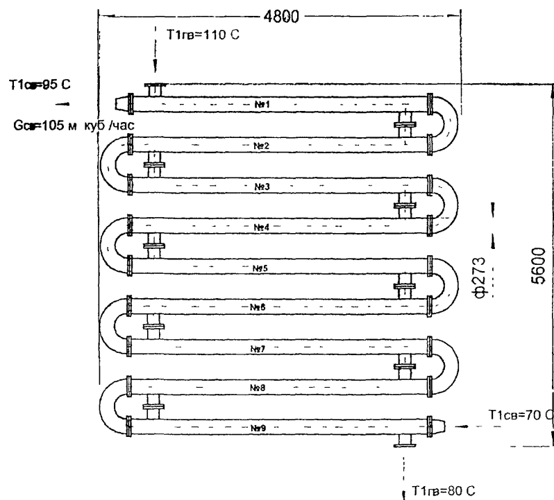
Масса блока- 4870кг.
