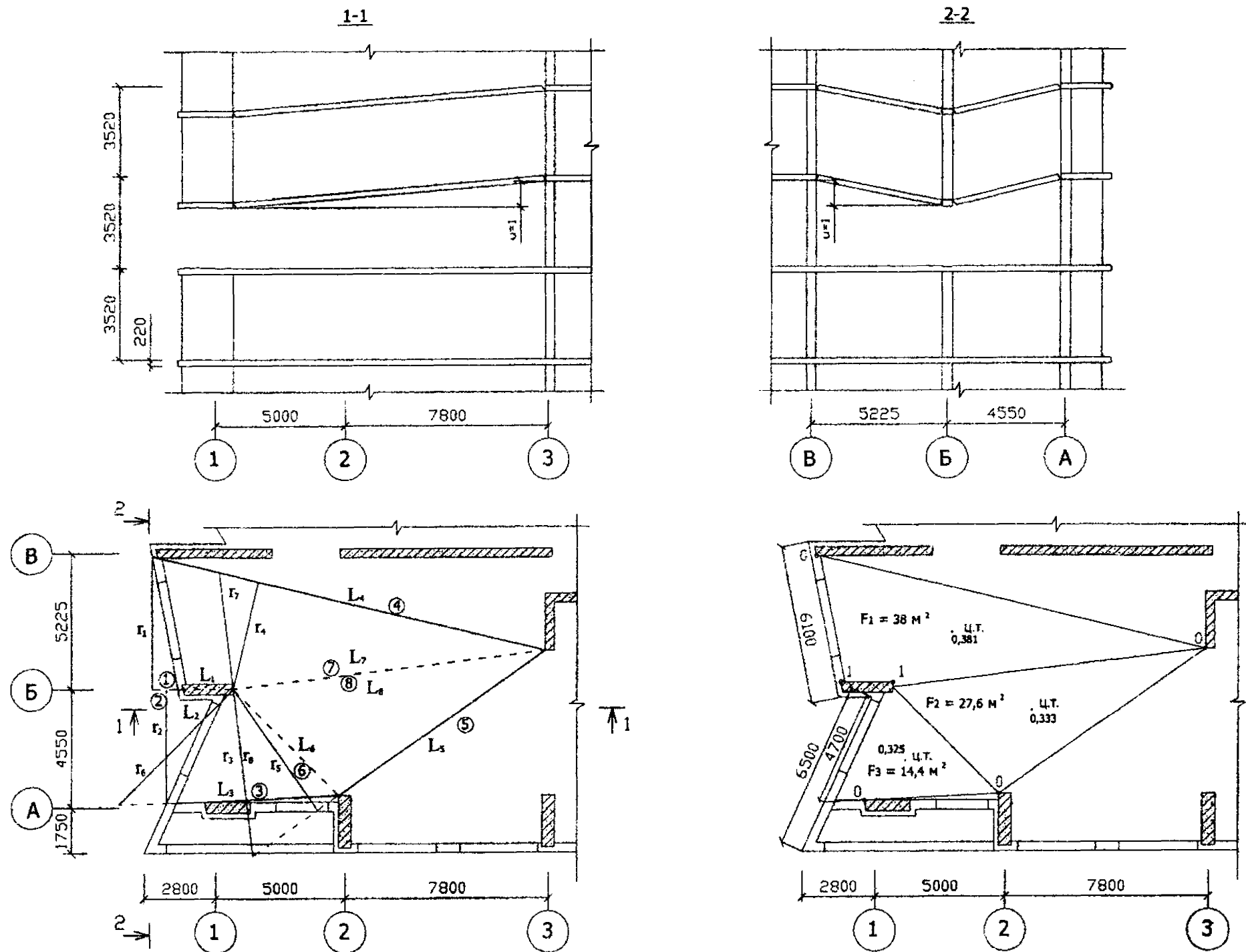
РИСУНОК А1.2 СХЕМА 1. МЕХАНИЗМ ОБРУШЕНИЯ ПЕРВОГО ТИПА.
