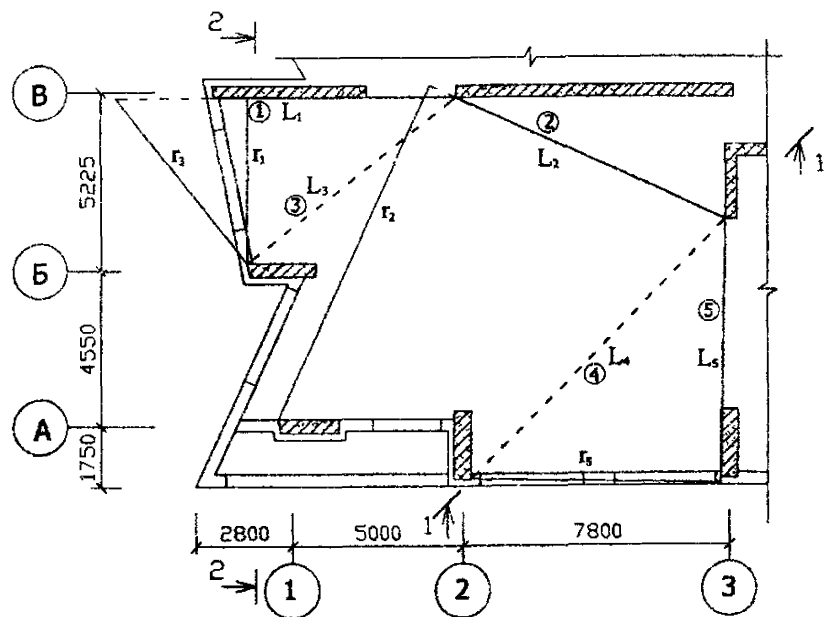
РИСУНОК А1.13 СХЕМА 3. МЕХАНИЗМ ОБРУШЕНИЯ ВТОРОГО ТИПА.
