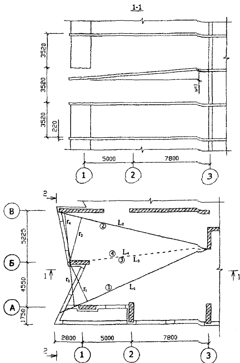
РИСУНОК А1.4 СХЕМА 1. МЕХАНИЗМ ОБРУШЕНИЯ ТРЕТЬЕГО ТИПА.
