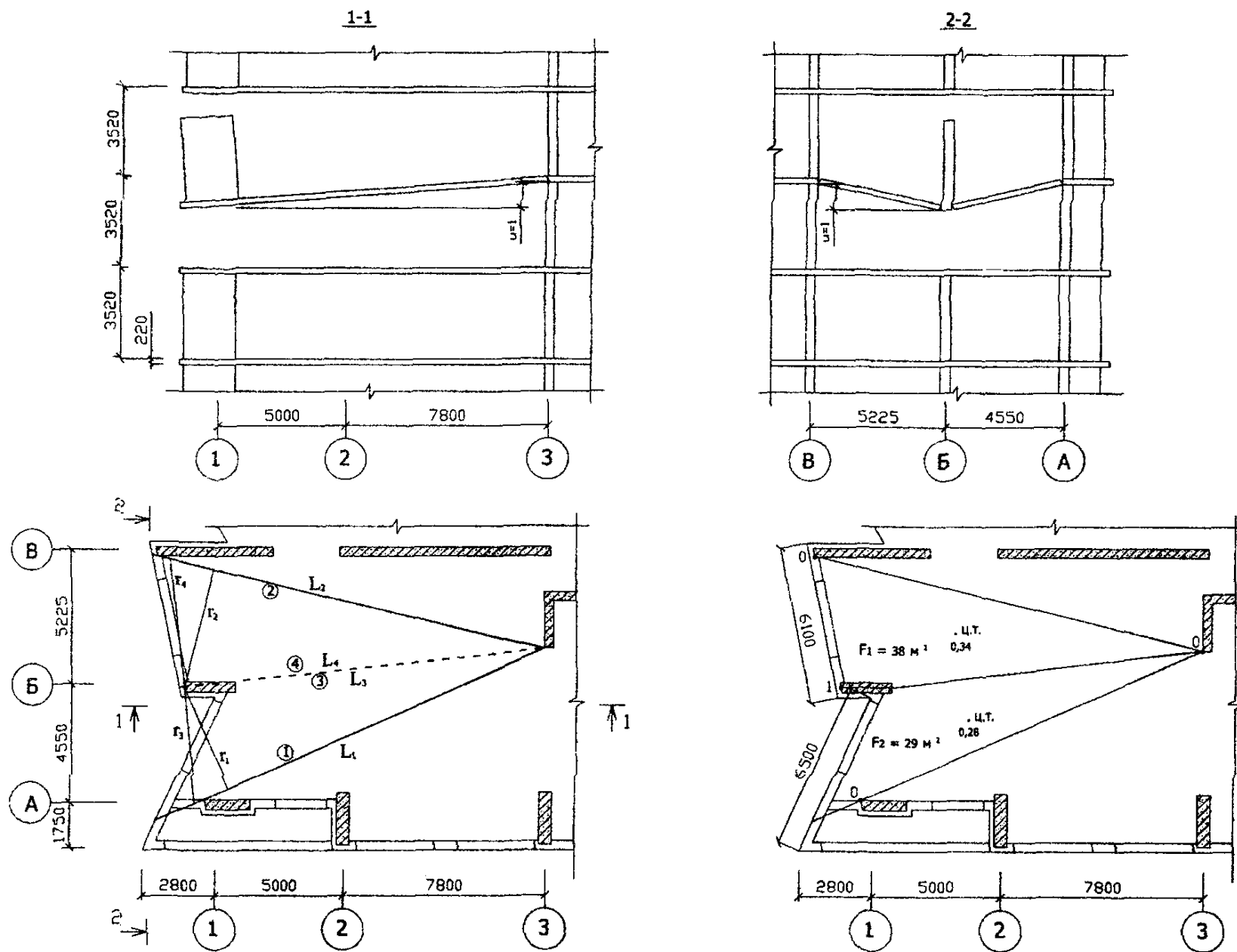
РИСУНОК А1.5 СХЕМА 1. МЕХАНИЗМ ОБРУШЕНИЯ ЧЕТВЕРТОГО ТИПА.
