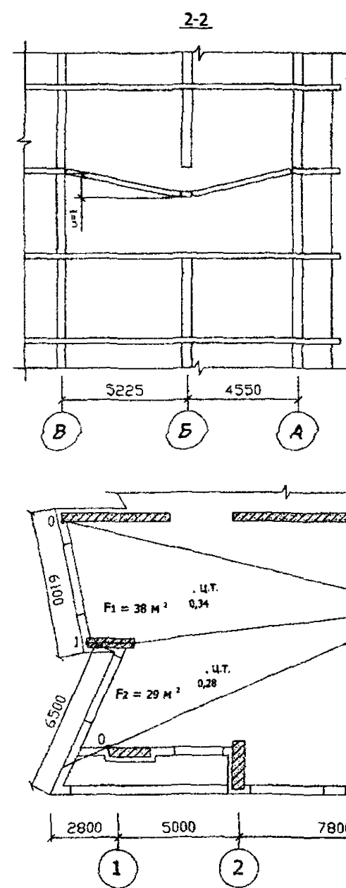
РИСУНОК А1.4 СХЕМА 1. МЕХАНИЗМ ОБРУШЕНИЯ ТРЕТЬЕГО ТИПА.
