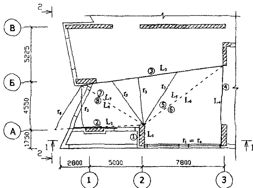
РИСУНОК А1.6 СХЕМА 2. МЕХАНИЗМ ОБРУШЕНИЯ ПЕРВОГО ТИПА.
