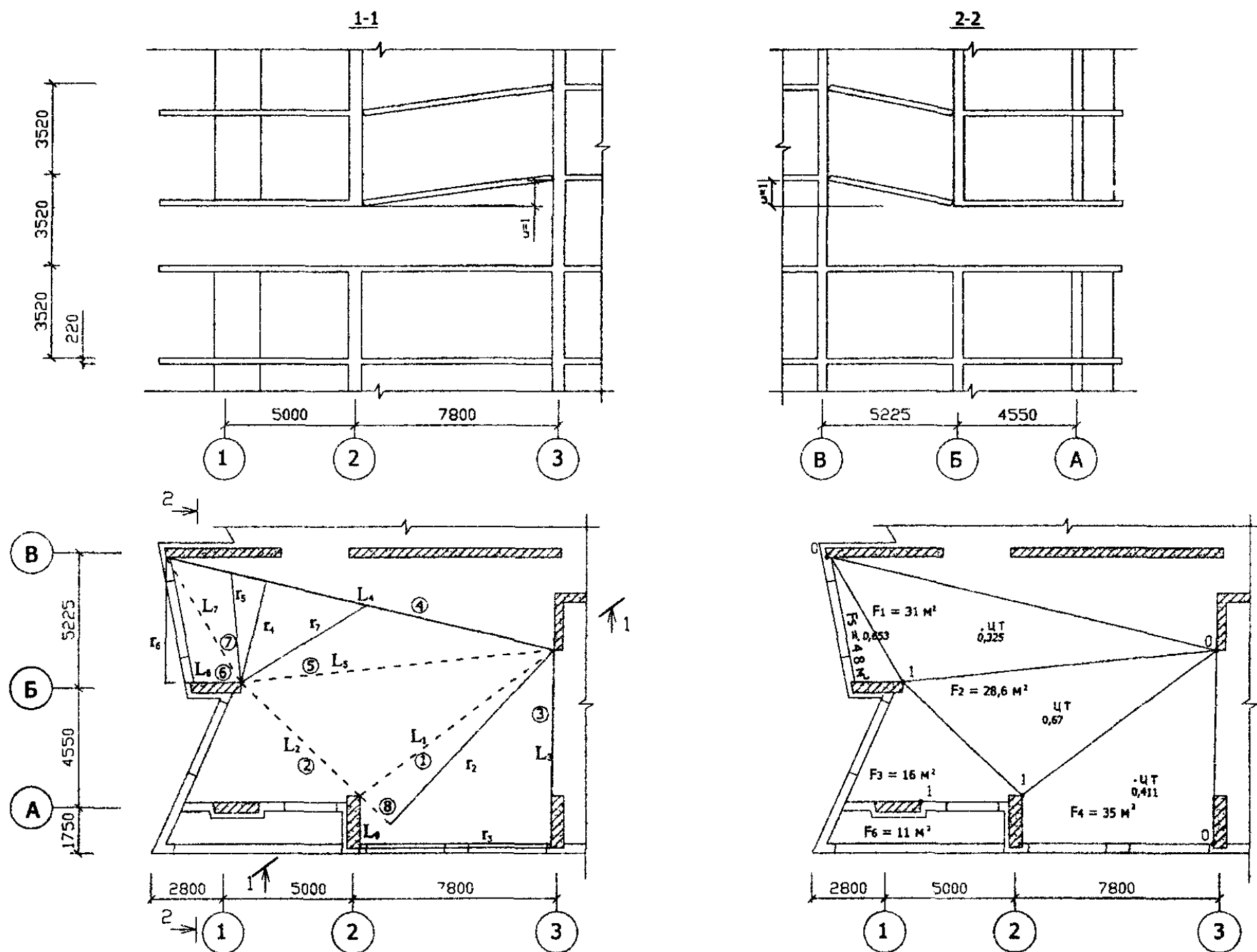
РИСУНОК А1 10 СХЕМА 1 ВАРИАНТ 1 МЕХАНИЗМ ОБРУШЕНИЯ ПЕРВОГО ТИПА.
