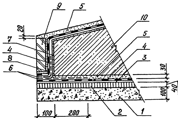
Рис. I2. Узел 8. Оклеечная гидроизоляция
