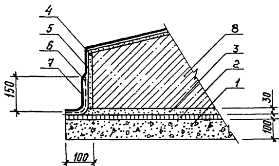
Рис. II. Узел 7. Литая и окрасочная гидроизоляция
