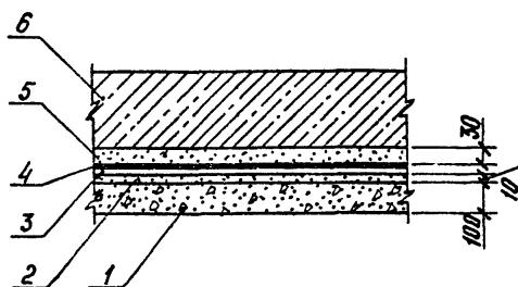
Рис. 5. Узел I. Окрасочная гидроизоляция
