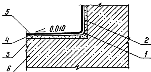
Рис. 13. Узел 9. Окрасочная гидроизоляция
