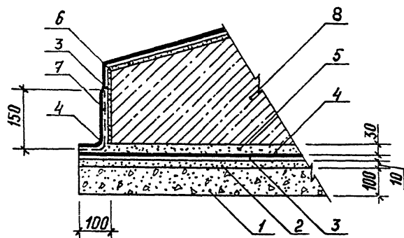
Рис. 9. Узел 5. Окрашенная гидроизоляция
