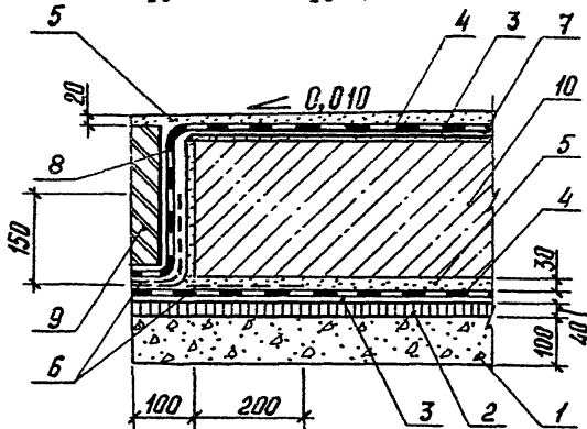
Рис. 20. Узел 16. Оклеенная гидроизоляция
