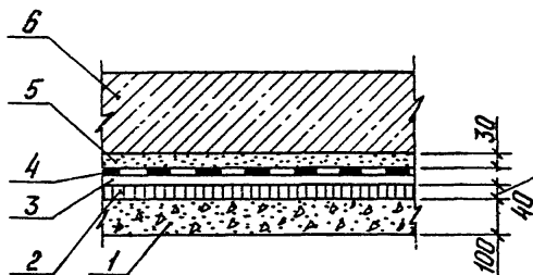
Рис. 8. Узел 4. Оклеечная гидроизоляция
