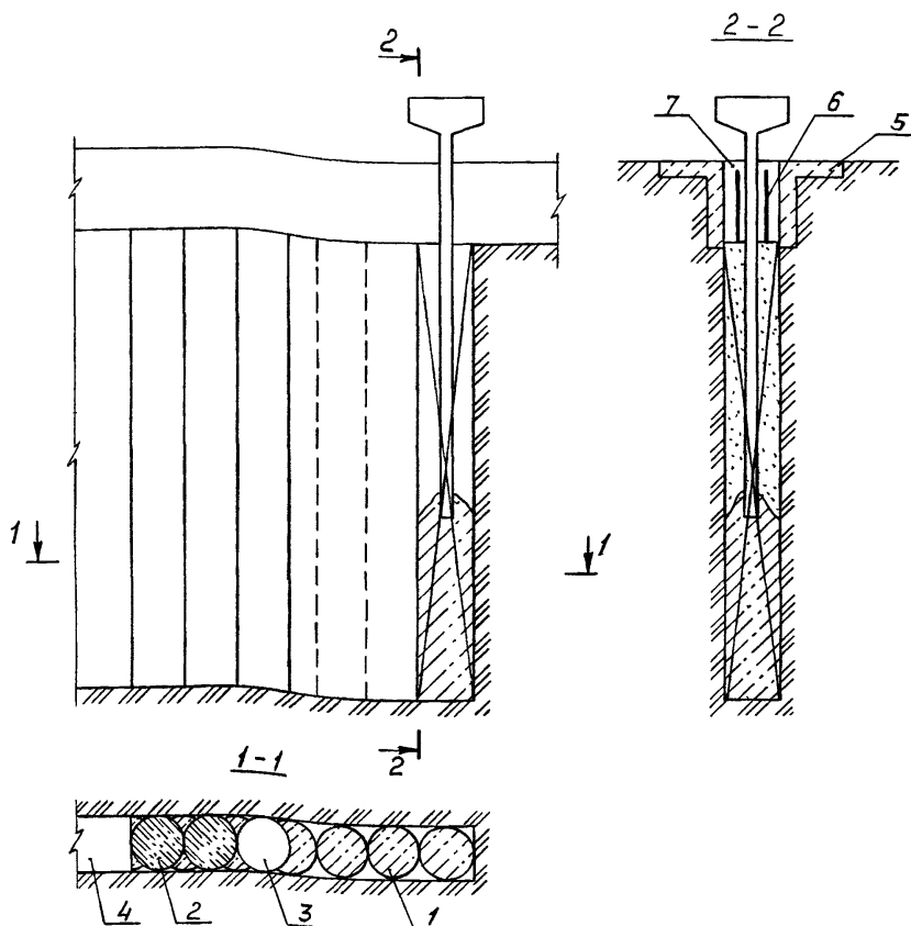
Рис.17. Схема производства работ при строительстве подземных сооружений способом "секущихся свай"
