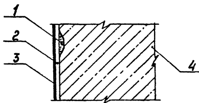
Рис. 23. Узел 19. Окрасочная гидроизоляция
