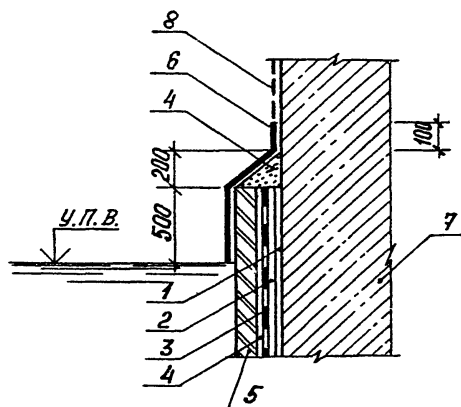
Рис. 16. Узел I2. Оклеечная гидроизоляция
