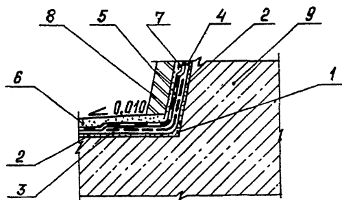
Рис. 22. Узел I8. Оклеенная гидроизоляция
