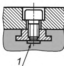
Рисунок В.6 — Правильное расположение гайки и болта
