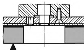
Рисунок 3 — Торцевое шлифование кольцевым кругом
