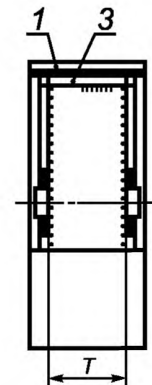
1 — основное ограждение; 3 — внутреннее ограждение
