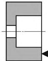
Рисунок 2 — Торцевое шлифование
