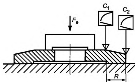
Рисунок В.3 — Испытательное оборудование
