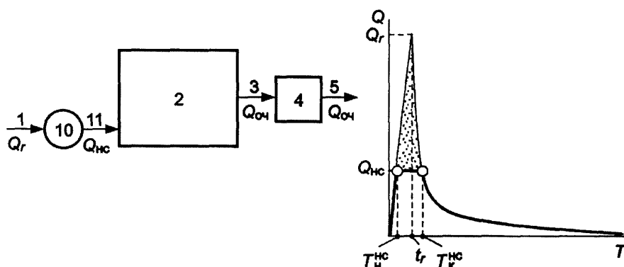
Рис. 1. Схема перекачки полного объема незарегулированного дождевого стока
