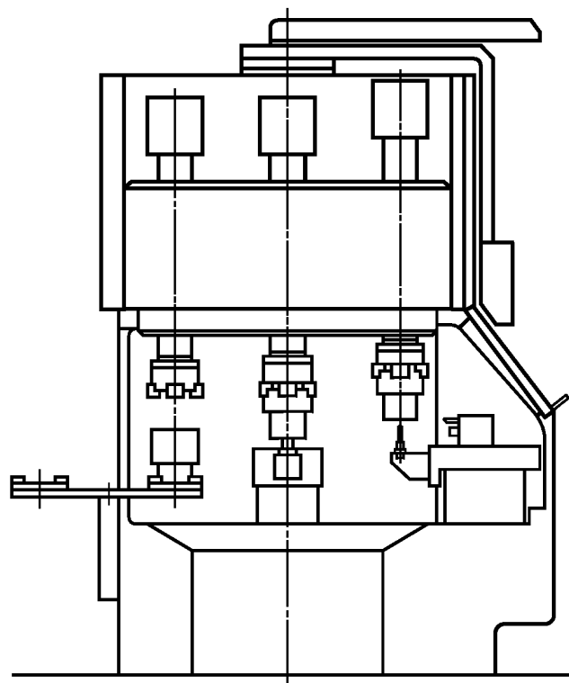
с) Пример вертикального многошпиндельного патронного токарного автомата с ЧПУ
