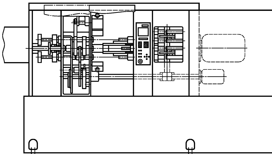
б) Пример многошпиндельного пруткового кулачкового токарного автомата
