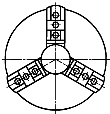
Рисунок 2 — Зажимной патрон
