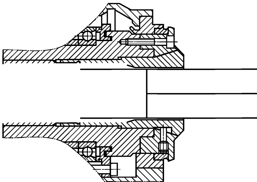
Рисунок 3 — Зажимная цанга
