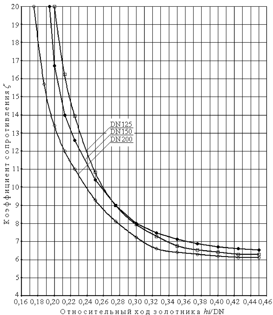
Рисунок 7 - Зависимости коэффициентов сопротивления от относительного хода золотника \zeta = f\left(\frac{h_i}{DN}\right) для клапанов DN 125, 150, 200
