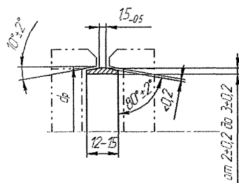
Рисунок 2 Коническое подкладное кольцо
