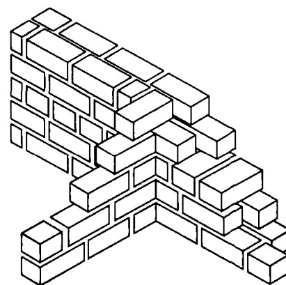
Рисунок 6.4в – Сопряжение наружной кладки толщиной в 2 однотипных блока и внутренней стены
