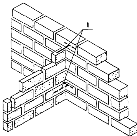
Рисунок 6.4б – Примыкание перегородки к стене
