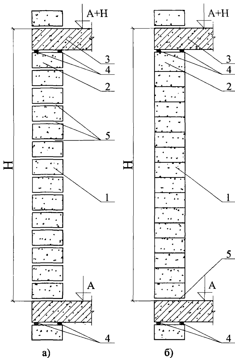
Рисунок 6.5 – Схема кладки наружных самонесущих с поэтажным опиранием стен из мелких ячеистобетонных блоков а) блоки на растворе; б) блоки на клею
