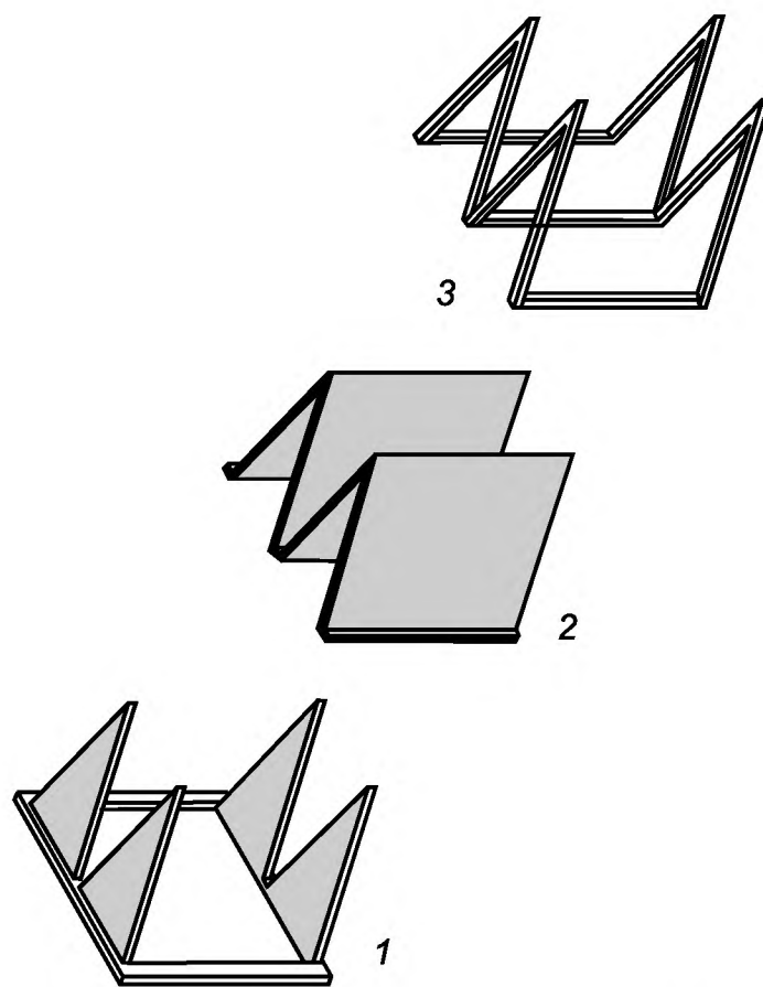
1 — W-форма рамки; 2 — фильтрующий материал; 3 — W-форма прижимной рамки
