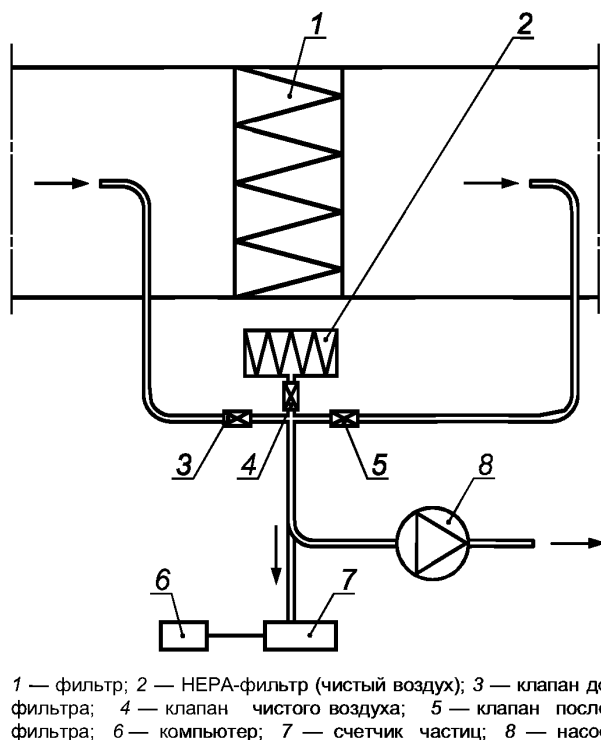
Рисунок 5 — Схема системы отбора проб аэрозоля
