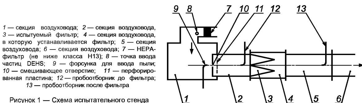
Рисунок 1 — Схема испытательного стенда
