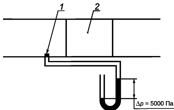
1 — закрытое отверстие отбора давления; 2 — секция испытательного устройства
