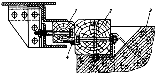
Рис. 4 Схема донного уплотнения
