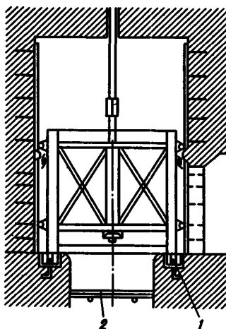
Рис. 8. Схема цилиндрического затвора
