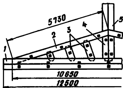
Рис 16. План королевской колоды
