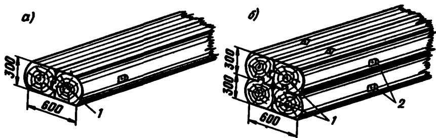
Рис. 17. Конструкции колод
