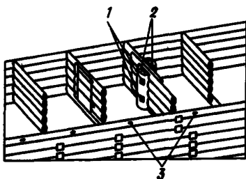
Рис. 18. Первый способ нарубки лицевых стен камеры шлюза
