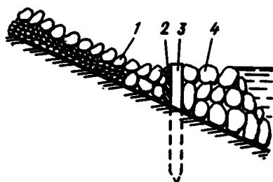
Рис. 13 Поперечный разрез заборки 1 — вымостка перед заборкой, 2 — пластина заборки, 3 — свая заборки; 4 — наброска за заборкой
