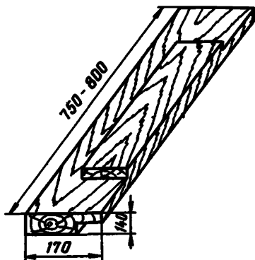
Рис. 12. Шпоночный вкладыш
