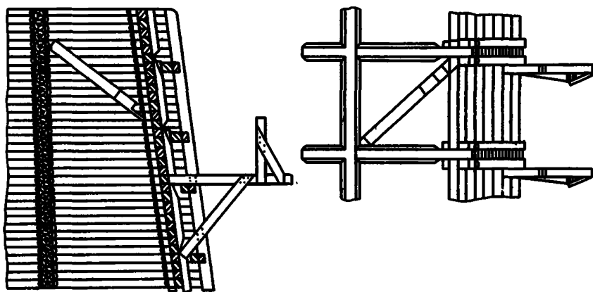
Рис. 29. Схема установки кронштейнов
