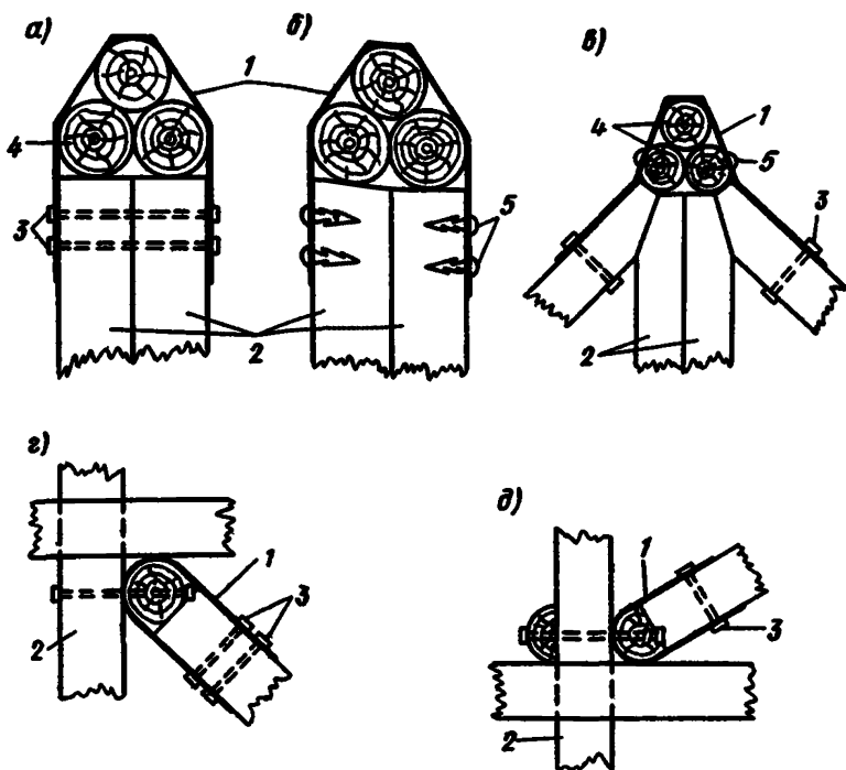
Рис. 26. Крепление хомута
