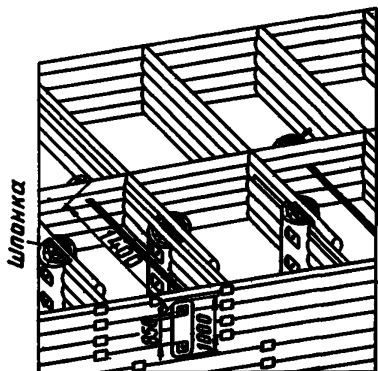
Рис. 19. Второй способ нарубки лицевых стен камеры шлюза
