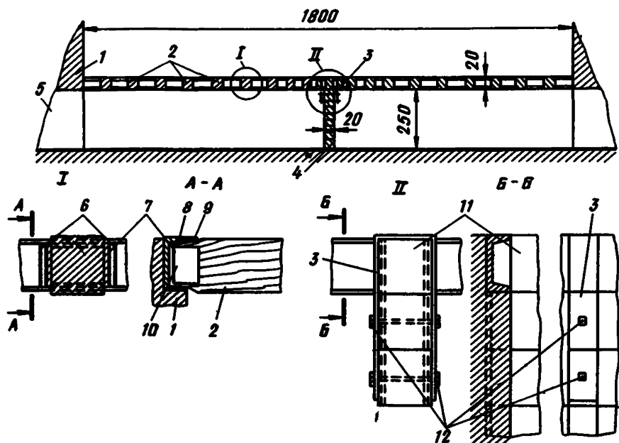
Рис. 10. Схема ниши гашения (разрезы)
