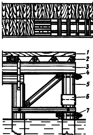
Рис 15. Схема поперечного настила
