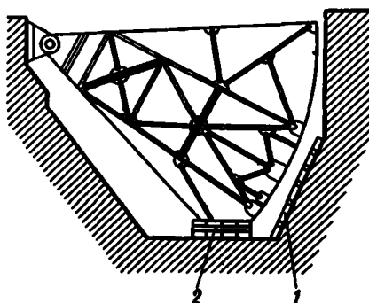
Рис 5. Схема рабочей зоны 1 — лестница; 2 — опорные клетки
