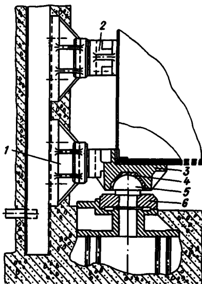
Рис. 2. Пятавое устройство ворот шлюза
