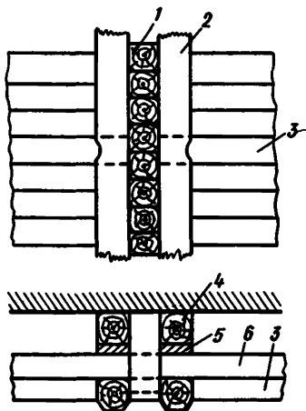
Рис. 22. Отбойная система, тип I
