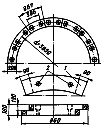
Рис. 9. Дубовое кольцо уплотнения
