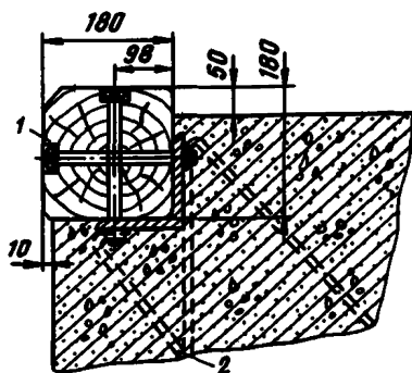
Рис. 7. Брус уплотнения порога короля 1 — брус уплотнения; 2 — анкерный болт
