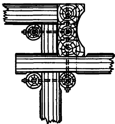
Рис. 14. Схема крепления веревяльного столба
