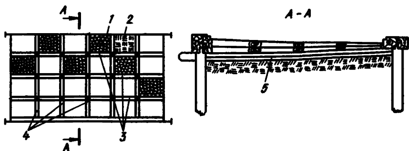
Рис. 24. Схема-ростверка
