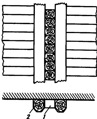
Рис. 23. Отбойная система, тип II
