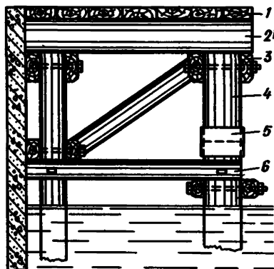
Рис. 28. Схема верхнего строения
