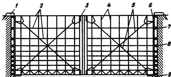
Рис 1 Схема двухстворчатых ворот шлюза
