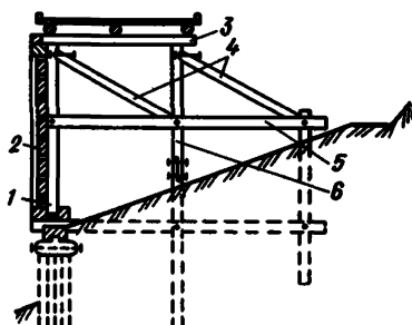
Рис. 27. Поперечный разрез эстакады
