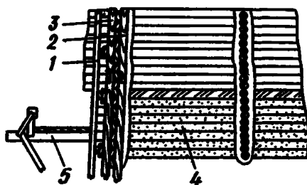
Рис. 20. Схема верхней части ряжевых стен шлюза
