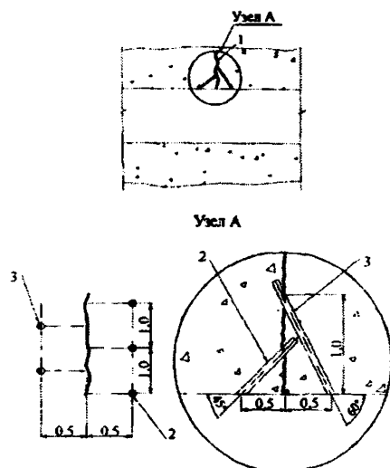
Рисунок Л.3.2 – Схема локализации угловых трещин (швов) с организацией сбора фильтрующей воды и последующим уплотнением инъецированием
