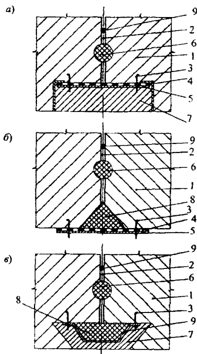
а - внешний компенсатор; б - шпонка на поверхности; в - шпонка внутри;
