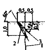
Рисунок Л.3.1 – Схемы расположения скважин при уплотнении фильтрующих трещин и швов
