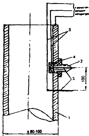
1 – труба стальная; 2 – свеча автомобильная; 3 – центральный электрод; 4 – изолятор; 5 – провод
