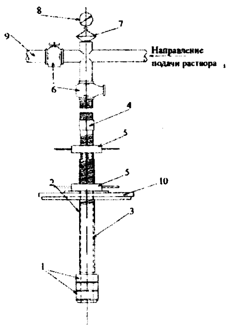
Рисунок Л.3.11 – Ликвидация точечного очага фильтрации (общий случай)
