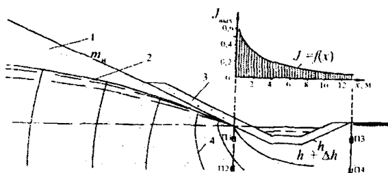
Рисунок Д.5 – Эпюра продольных деформаций гребня плотины
