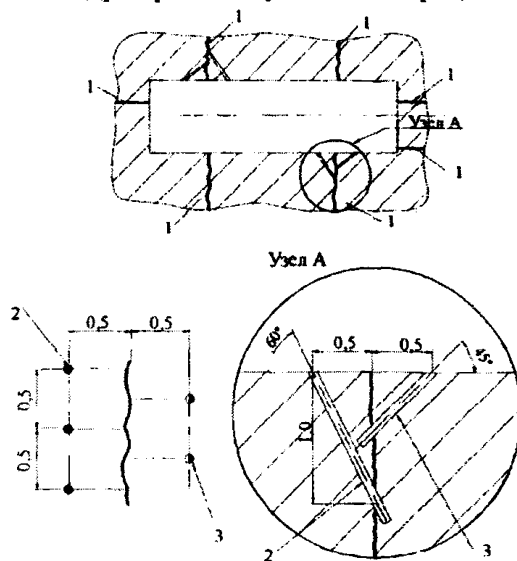
Рисунок Л.3.3 – Дренажное и уплотнение трещин инъекцией
