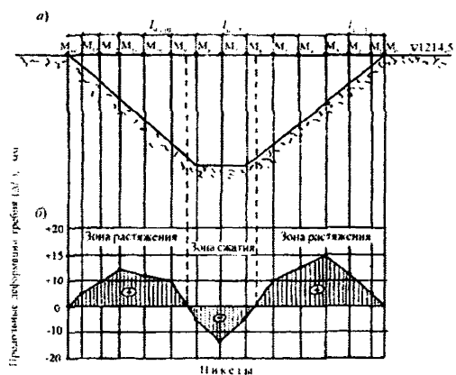
Рисунок Д.4 – График осадки гребня плотины
