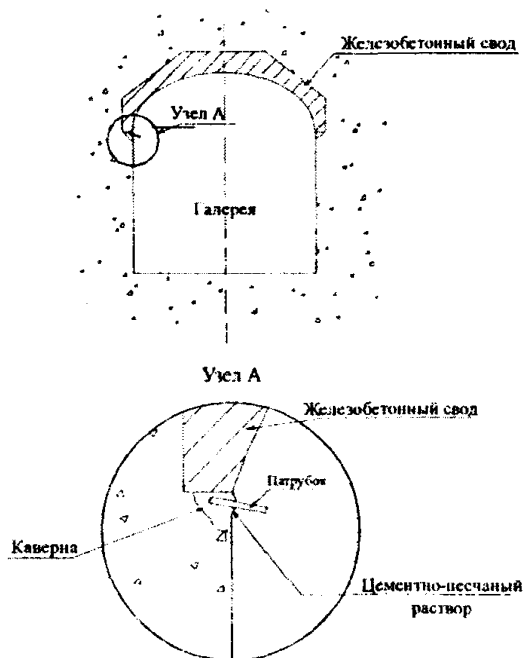
Рисунок Л.3.8 – Схема устройства дренажа в стыках стен со сводом
