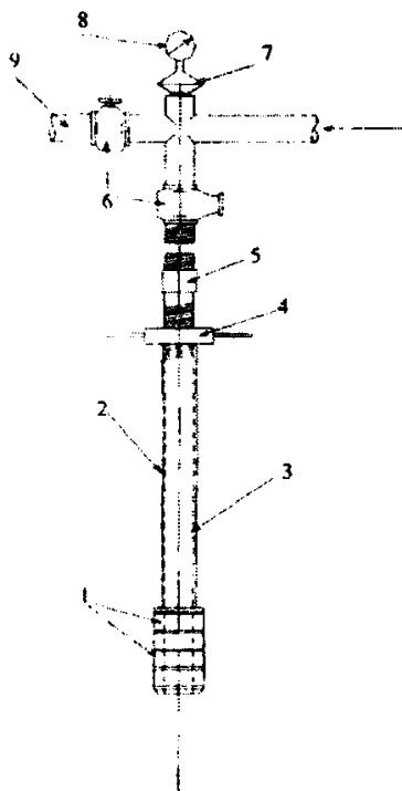
Рисунок Л.3.9 – Площадная инъекция бетона с использованием тампона (при наличии развитой дефектной зоны)
