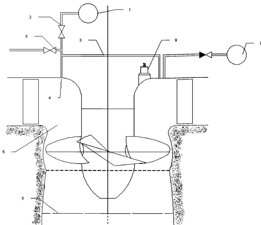
Рисунок В.1. Воздушная система отжатия воды из камеры рабочего колеса поворотно-лопастной гидротурбины: 1- Магистраль воздушной системы; 2- клапан пуска сжатого воздуха; 3-подводящий воздухопровод; 4-отверстия в крышке турбины; 5- камера рабочего колеса; 6- отжатый уровень воды; 7- устройство поддержания отжатого уровня; 8-клапан пуска атмосферного воздуха; 9- клапан срыва вакуума.
