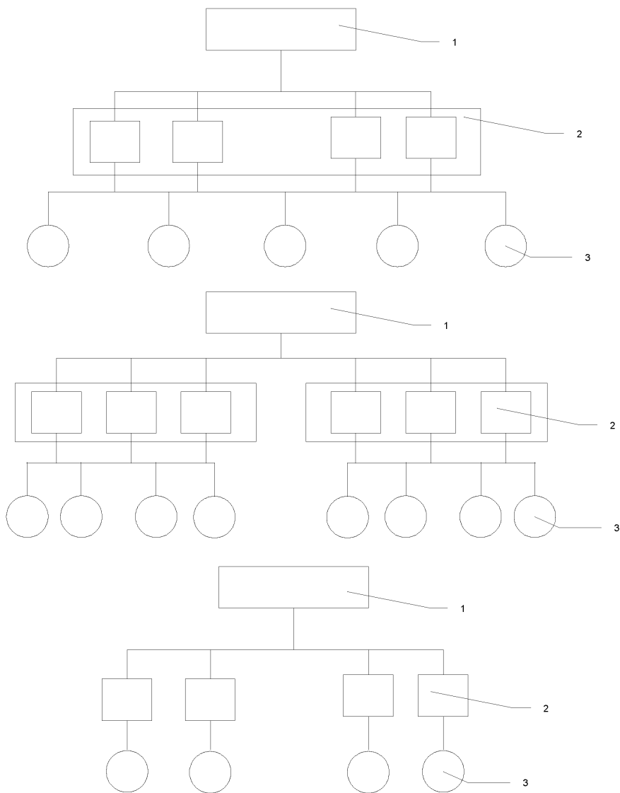
Рисунок В.5. Компоновка воздушной системы отапления: объединенные (общестанционные)- верхняя схема, групповые (блочные)- средняя схема и индивидуальные (агрегатные)- нижняя схема.
