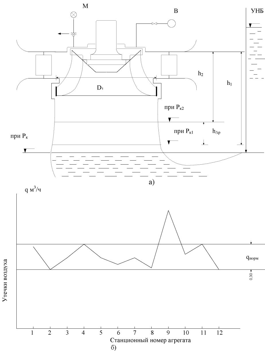
Рисунок В.4. Контроль утечки воздуха из камеры рабочего колеса турбины при работе в режиме СК:
