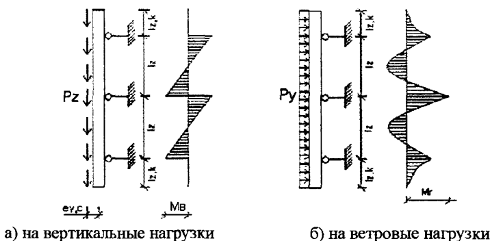
Рисунок 14 - Расчетные схемы вертикальной направляющей.
