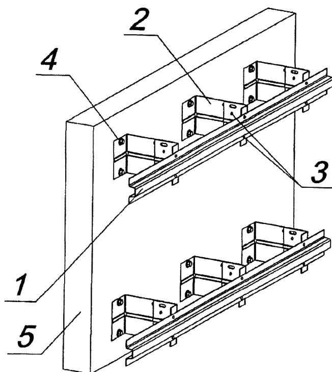
1 – профиль шляпный 23 (60); 2 – кронштейн составной; 3 – заклепки (самонарезающие винты); 4 – анкер; 5 – стена.
