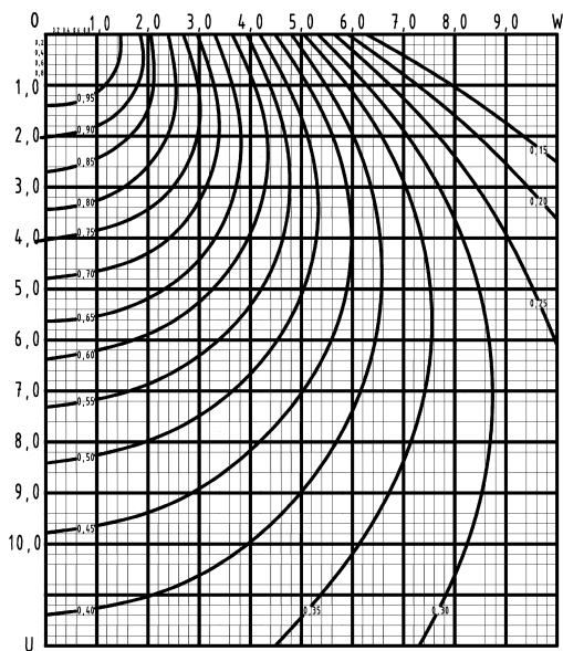
Рис. П.Е.10 Графики значений \alpha_1 = \frac{\sigma_1}{p_0} при \frac{2a}{B} = 6
