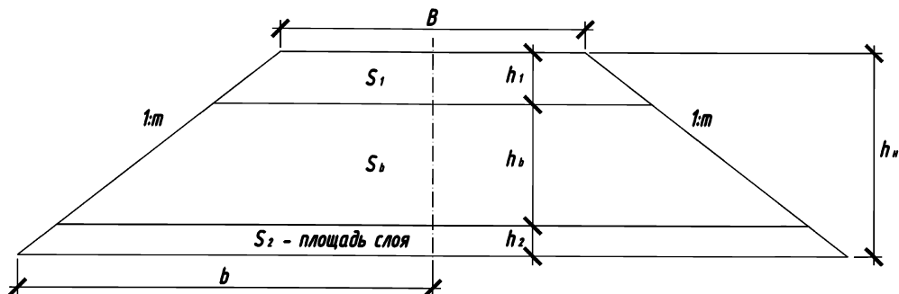
Рис. 20 Расчетная схема
