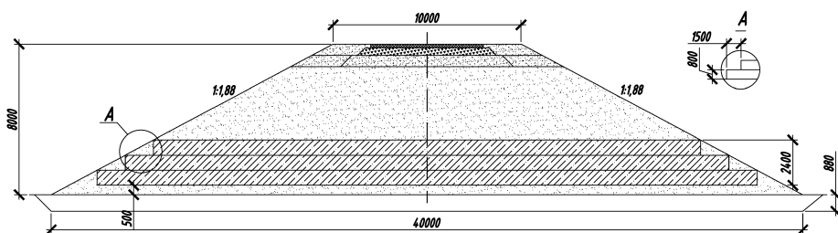
Рис. 22 Конструкция легкой насыпи на расчетном поперечнике
