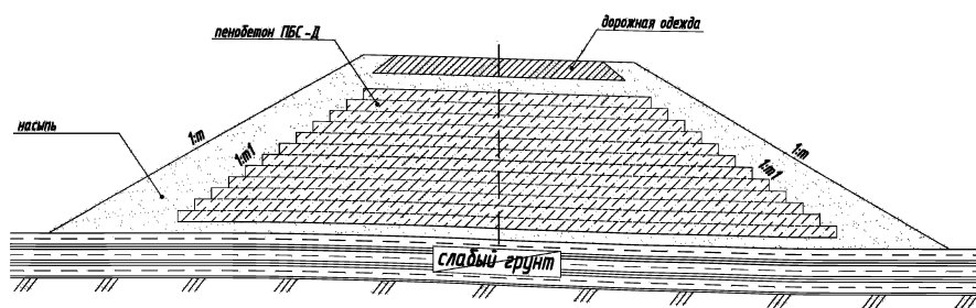
Рис. 1 Легкая насыпь
