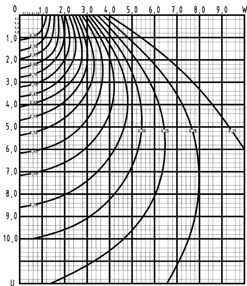
Рис. П.Е.8 Графики значений \alpha_1 = \frac{\sigma_1}{p_0} при \frac{2a}{B} = 3
