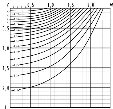
Рис. П.Е.7 Графики значений \alpha_2 = \frac{\sigma_2}{p_0} при \frac{2a}{B} = 1,6
