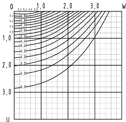
Рис. П.Е.9 Графики значений \alpha_2 = \frac{\sigma_2}{p_0} при \frac{2a}{B} = 3
