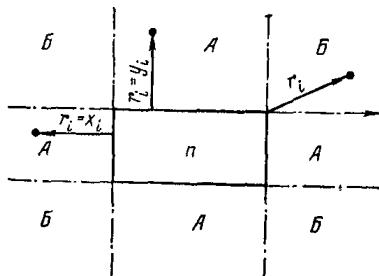
Рис. 27. Взаимное расположение зон основания, примыкающих к фундаментной плите
