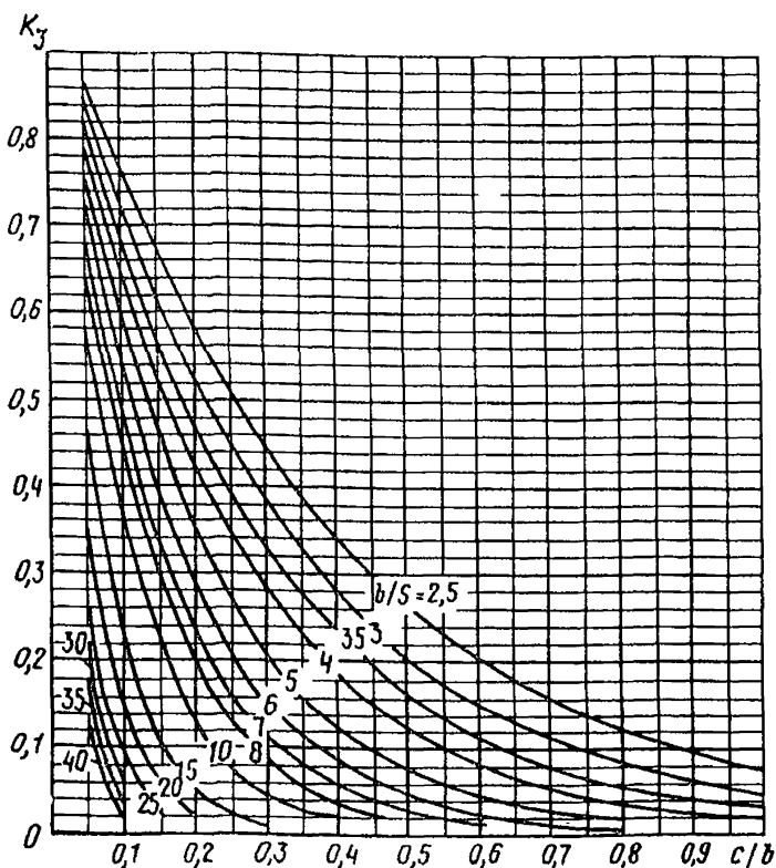
Рис. 39. График для определения коэффициента K_z в зависимости от c/b и b/s
