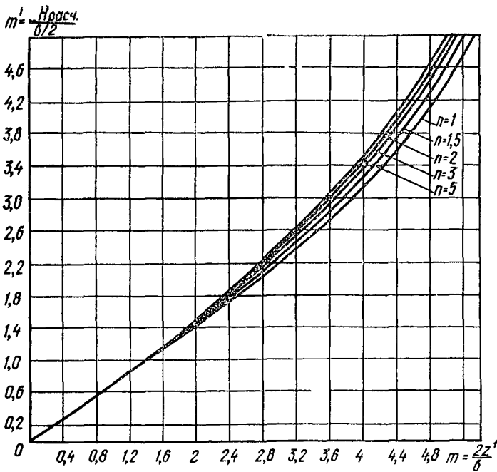
Рис. 6. График для определения толщины сжимаемого слоя H , эквивалентного по осадке условно органической части полупространства глубиной z' , при заданном отношении сторон фундаментной плиты n
