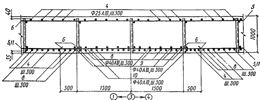
Рис. 56. Сечение 2—2 плиты, показанное на рис. 46—51
