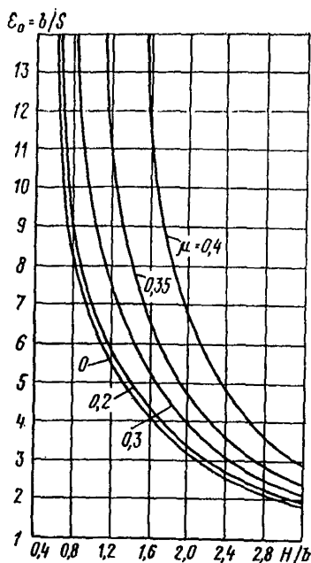
Рис. 24. Зависимость параметра \varepsilon_0 от H/b и \mu при n \rightarrow \infty
