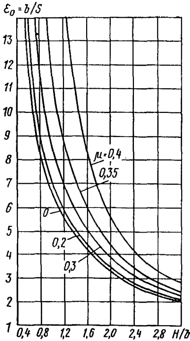
Рис. 22. Зависимость параметра \epsilon_0 от H/b и \mu при n=3
