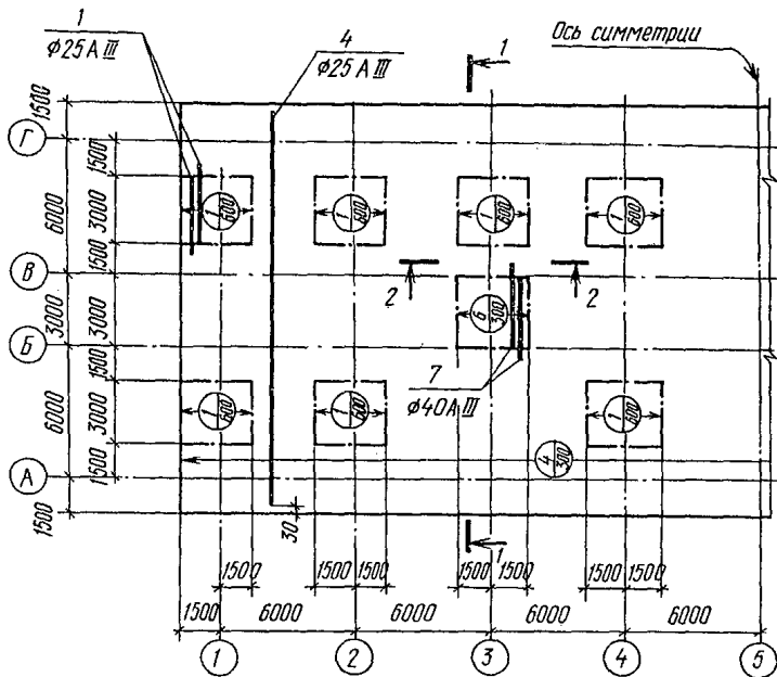
Рис. 51. План раскладки арматуры второго слоя верхней зоны
