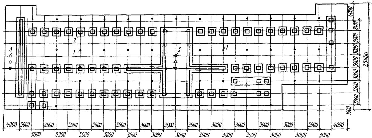
Рис. 18. Схема расположения осадочных марок на плане фундаментной плиты многоэтажного административного здания (стенные марки показаны условно)
