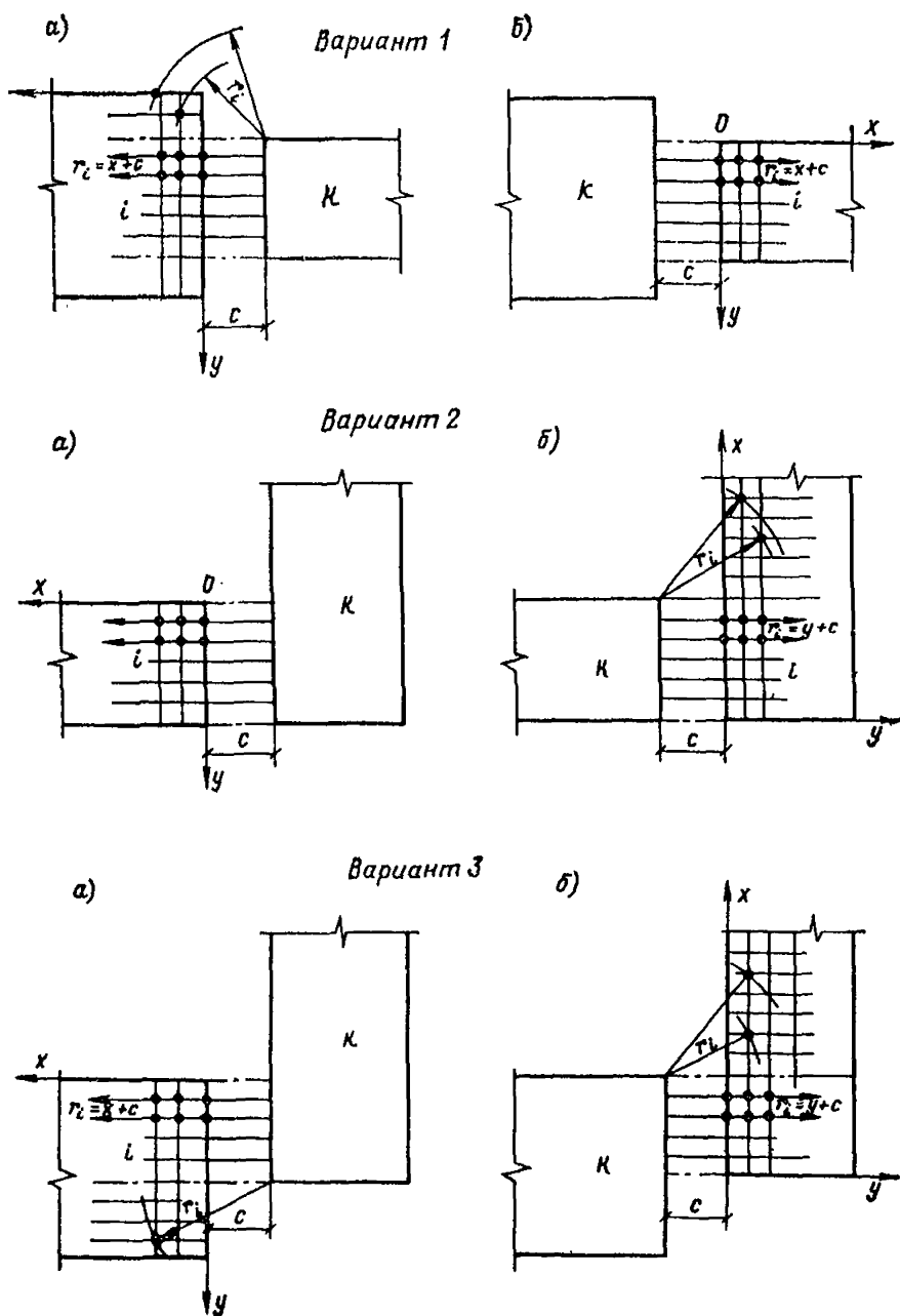
Рис. 28. Схема относительного расположения фундаментных плит (варианты 1—3)
