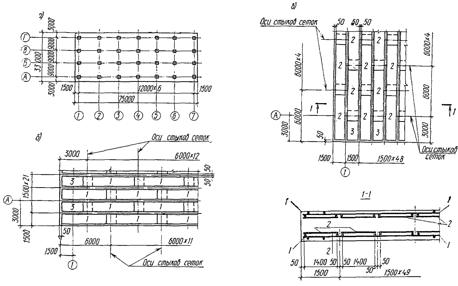
Рис. 17. Схема раскладки унифицированных сеток армирования прямоугольной плиты
