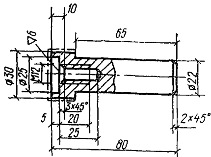
Рис. 66. Корпус стеной марки
