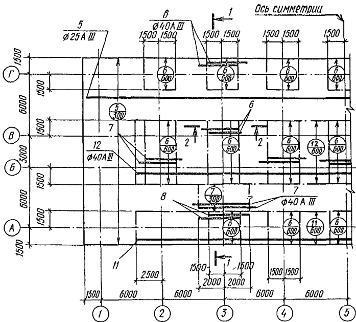
Рис. 47. План раскладки арматуры второго слоя нижней зоны
