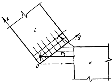
Рис. 29. Схема относительного расположения фундаментных плит (варианты 4, 5)
