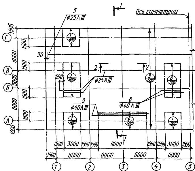
Рис. 50. План раскладки арматуры первого слоя верхней зоны
