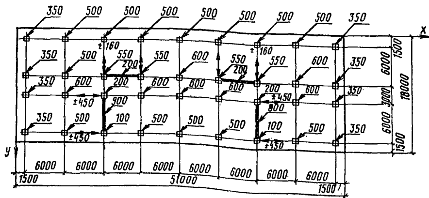
Рис. 42. Схема нагрузок, передаваемых на фундаментную плиту колоннами каркаса и диафрагмами жесткости 16-этажного здания
