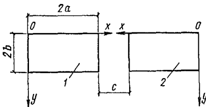
Рис. 26. Схема двух соосно расположенных однотипных фундаментных плит
