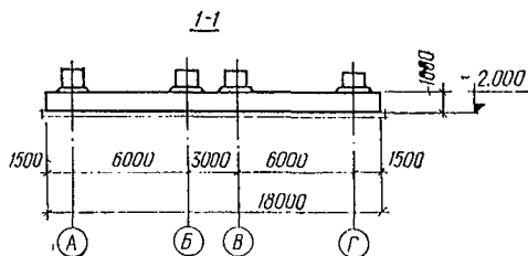
Рис. 45. Опалубка фундаментной плиты
