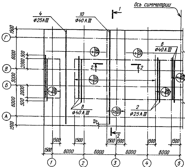
Рис. 46. План раскладки арматуры первого слоя нижней зоны
