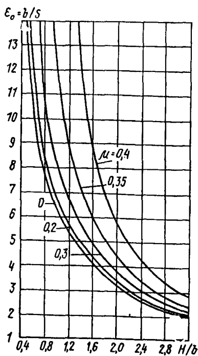
Рис. 23. Зависимость параметра \varepsilon_0 от H/b и \mu при n=5
