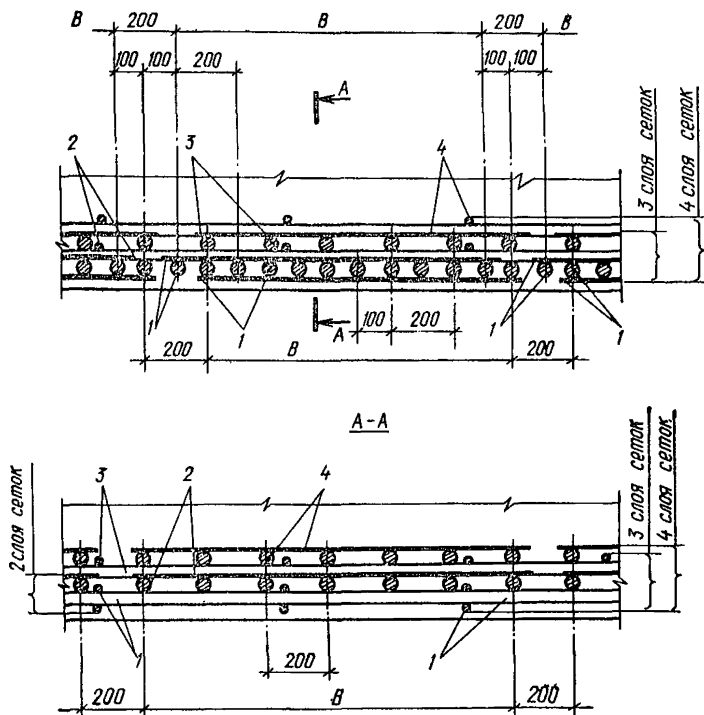
Рис. 16. Многослойное армирование плиты унифицированными сетками при шаге рабочих стержней нижней сетки 100 мм
