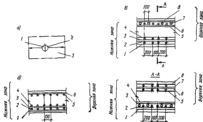
Рис. 65. Детали раскладки арматурных изделий
