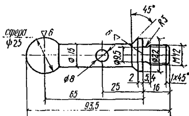
Рис. 68. Шаровой болт для геодезических работ
