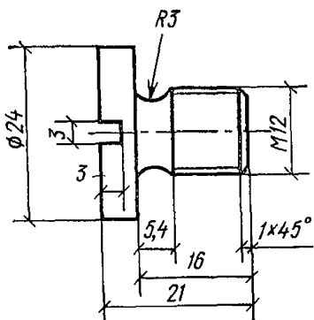
Рис. 67. Крышка стеной марки
