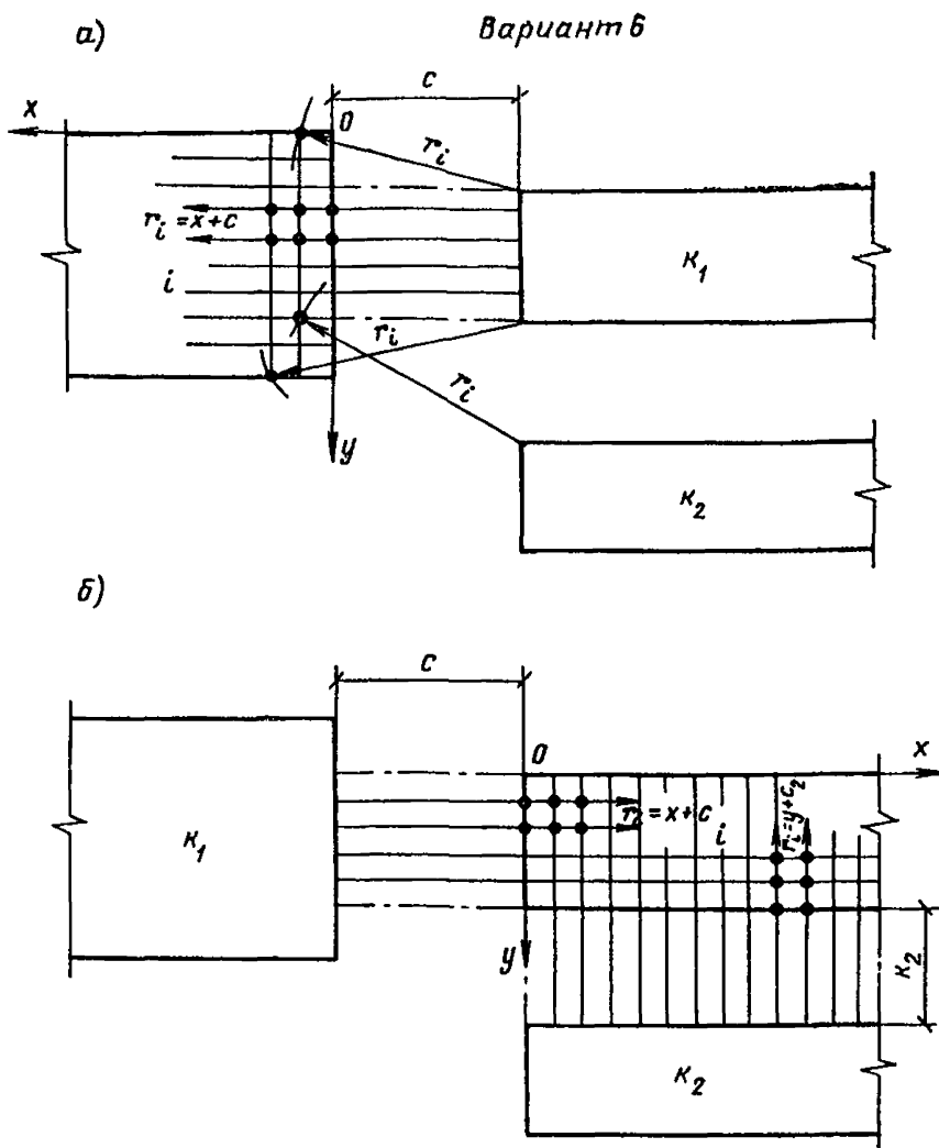
Рис. 30. Схема относительного расположения фундаментных плит Вариант б — параллельное и угловое расположение плит k_1 , k_2 ; i — K(x, y) определяются в прямоугольной и угловой зонах влияния; б — K(x, y) определяются в прямоугольных зонах влияния; i — рассчитываемая плита; k — влияющая плита
