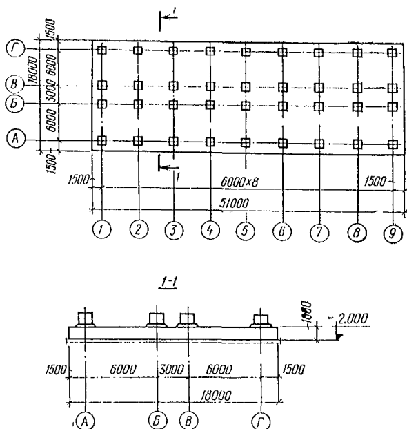
Рис. 45. Опалубка фундаментной плиты
