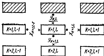
Рис. 36. Нагруженный участок расположен сверху от ненагруженного
