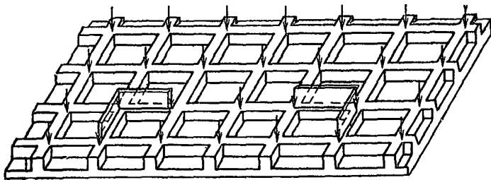
Рис. 14. Расчетная схема ребристой плиты
