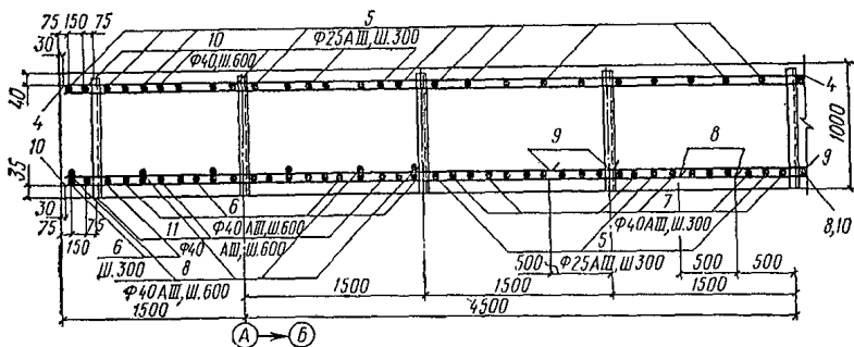
Рис. 53. Сечение 1—1 плиты (участок 1 на рис. 52)
