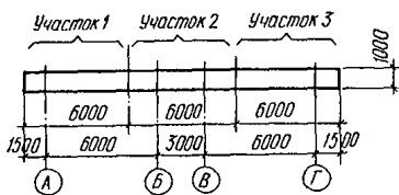
Рис. 51. План раскладки арматуры второго слоя верхней зоны
