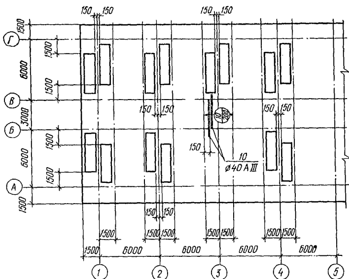
Рис. 61. План раскладки унифицированных сеток и арматуры второго слоя верхней зоны (верхние сетки)
