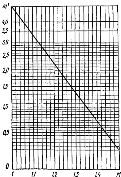
Рис. 3. График для определения коэффициента M в формуле (12)
