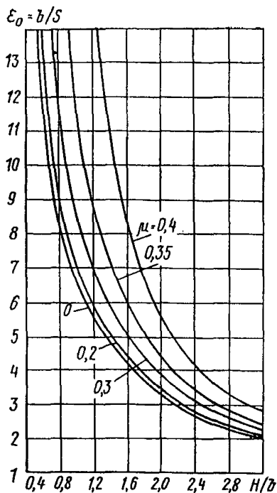
Рис. 22. Зависимость параметра \varepsilon_0 от H/b и \mu при n=3
