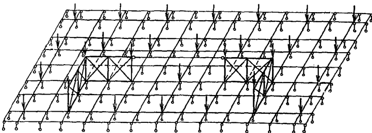
Рис. 12. Упрощенная расчетная схема совместного расчета плиты и связевого каркаса (стержневая пространственная система)
