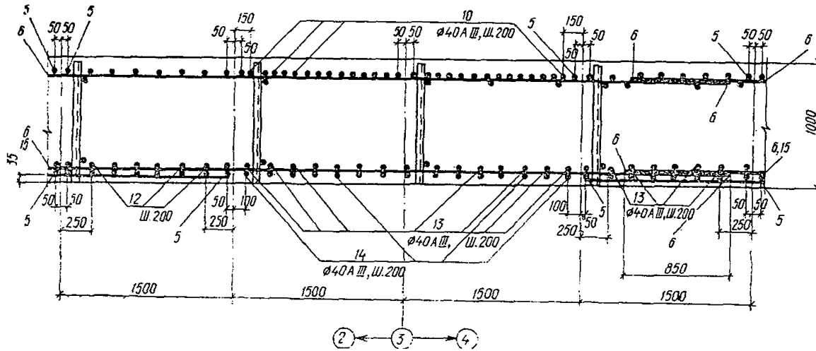
Рис. 64. Сечение плиты 1—1 на рис. 57—63
