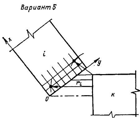
Рис. 29. Схема относительного расположения фундаментных плит (варианты 4, 5)
