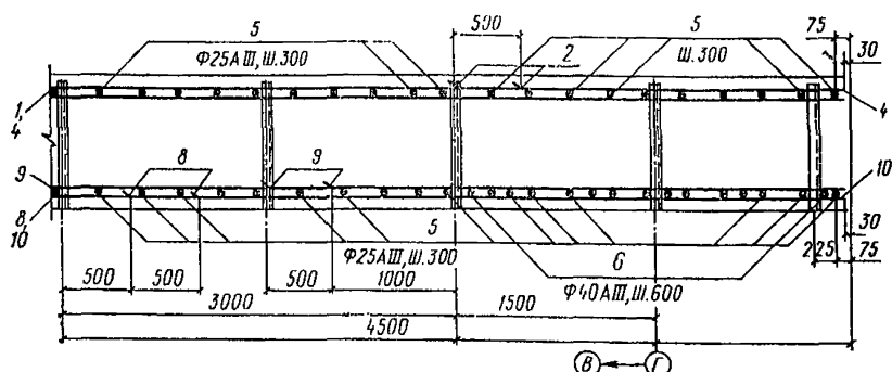
Рис. 55. Сечение 1—1 плиты (участок 3 на рис. 52)
