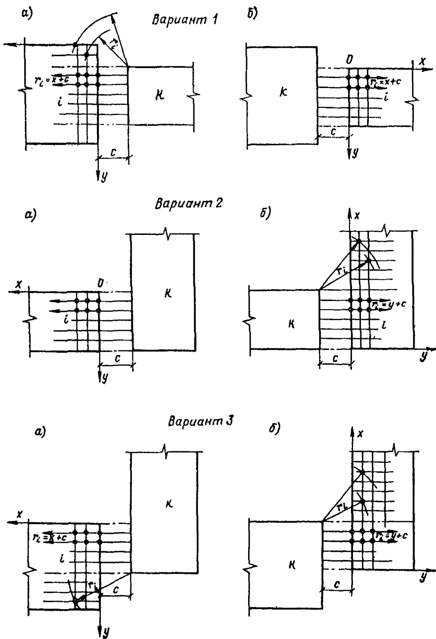
Рис. 28. Схема относительного расположения фундаментных плит (варианты 1—3)
