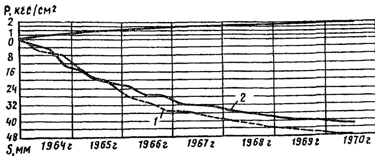
Рис. 19. Графики роста во времени измеренных осадков марок и среднего давления на грунт
