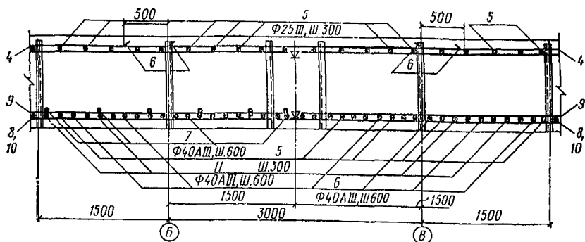
Рис. 54. Сечение 1—1 плиты (участок 2 на рис. 52)
