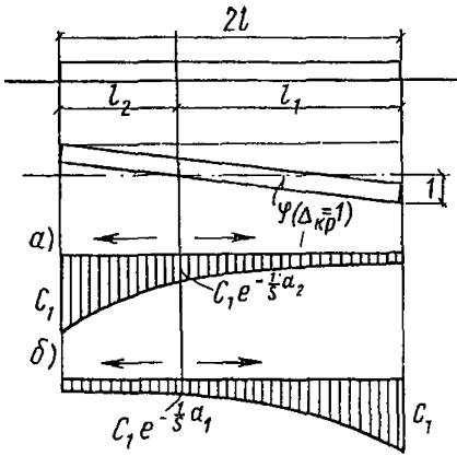
Рис. 41. Эпиюры компонент коэффициентов жесткости основания фундаментной плиты от влияния примыкающих зон а — слева; б — справа
