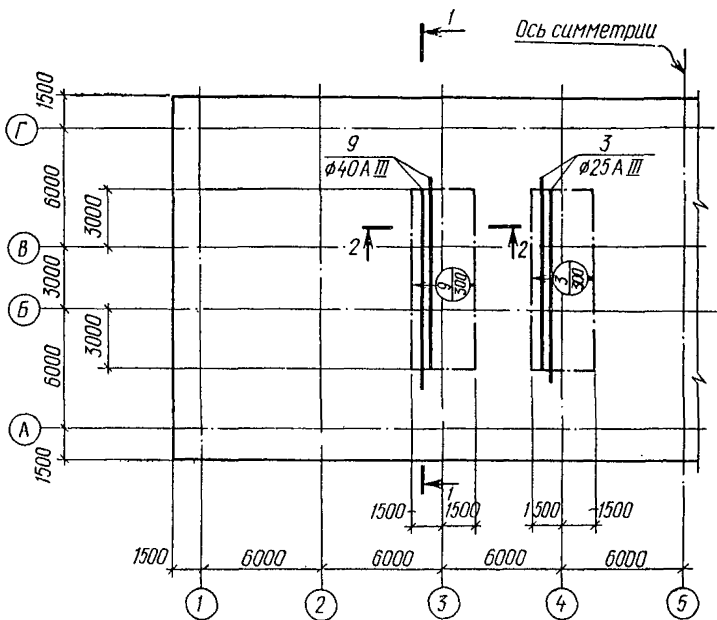
Рис. 48. План раскладки арматуры третьего слоя нижней зоны
