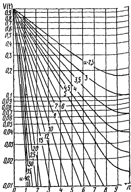
Рис. 25. График функции V(t) в зависимости от n и u
