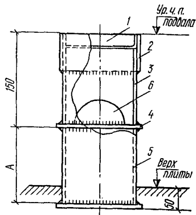
Рис. 69. Плитная марка
