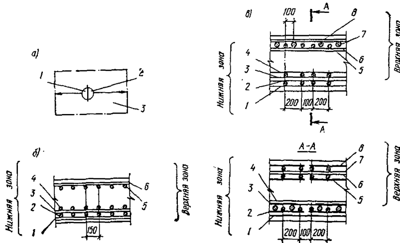
Рис. 65. Детали раскладки арматурных изделий
