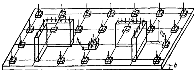
Рис. 8. Расчетная схема плиты ступенчато-переменной толщины, нагруженной вертикальными нагрузками, равномерно распределенными по отдельным прямоугольным площадкам
