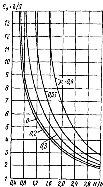
Рис. 24. Зависимость параметра \epsilon_0 от H/b и \mu при n \rightarrow \infty
