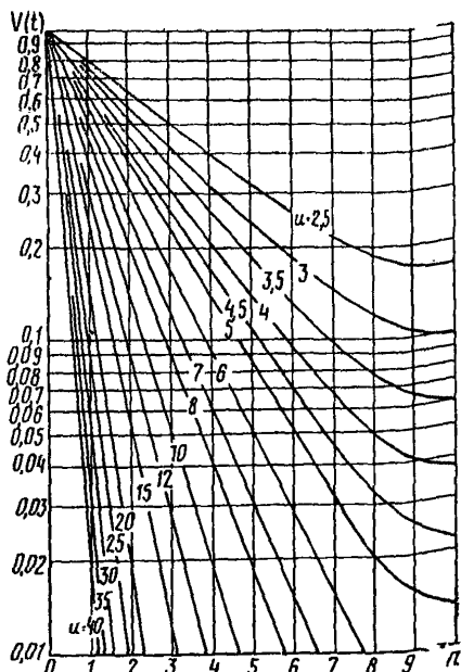
Рис. 25. График функции V(t) в зависимости от t и u
