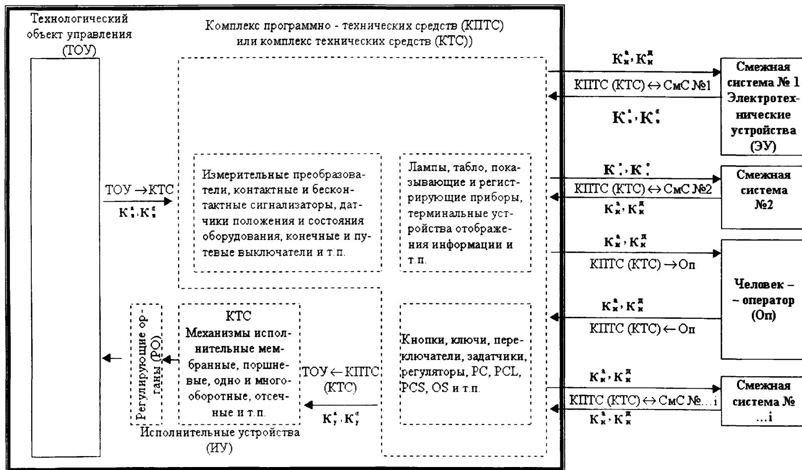
Схема автоматизированного технологического комплекса (АТК)
