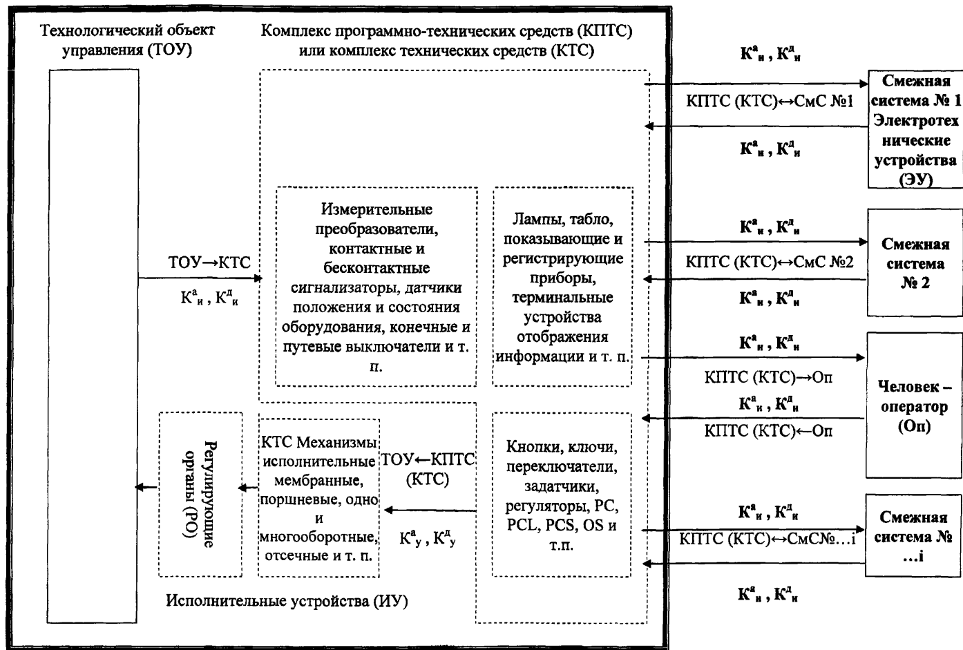
Схема автоматизированного технологического комплекса (АТК)
