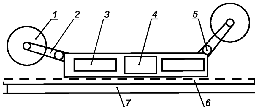
1 — шнек с резцами; 2 — поворотный редуктор; 3 — отделение редуктора; 4 — взрывозащищенное распределительное устройство; 5 — взрывозащищенный шнековый электродвигатель; 6 — расположение ременной передачи; 7 — забойный скребковый конвейер
