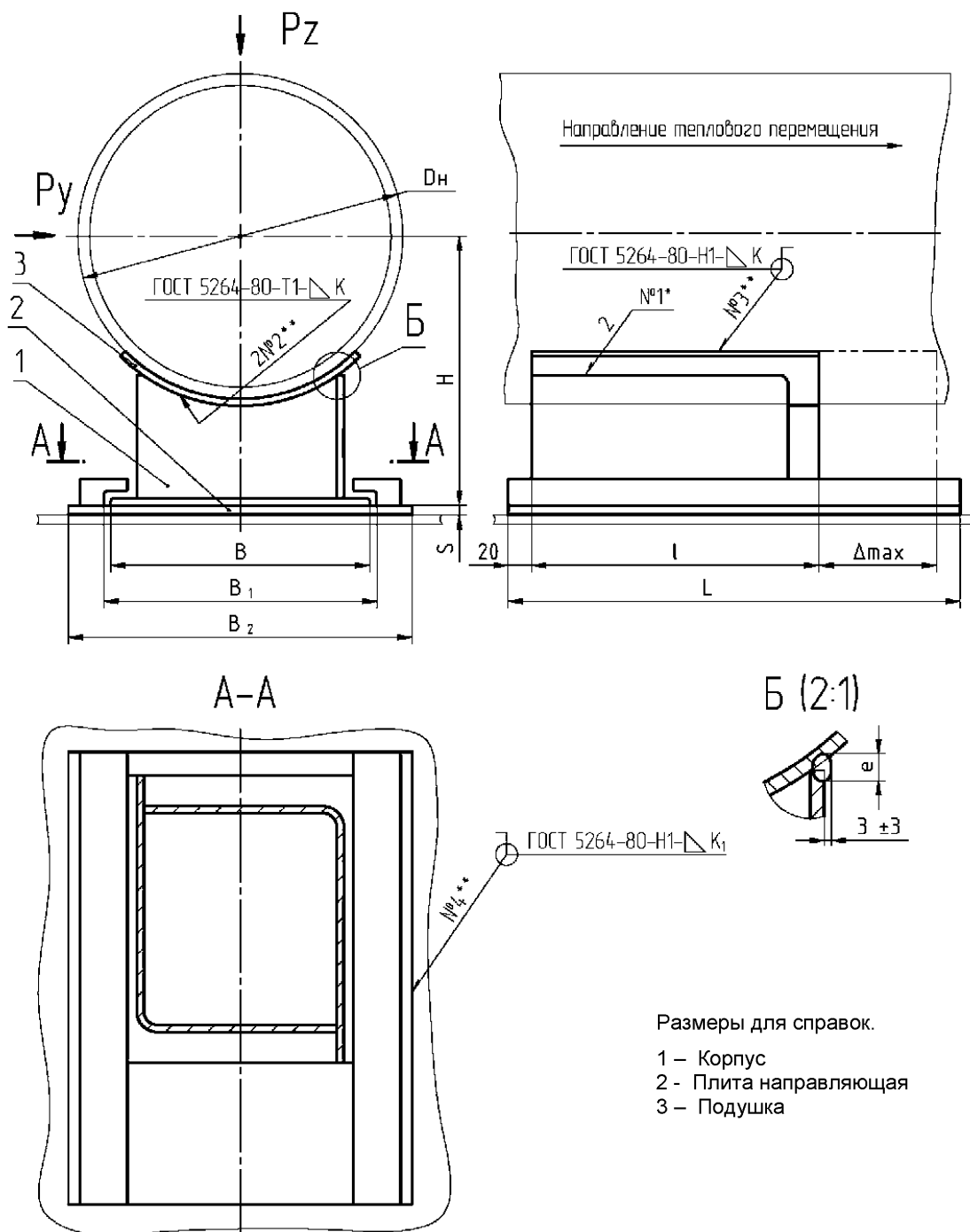
Рисунок 3 – Опора сварная направляющая для DN от 50 до 1600
