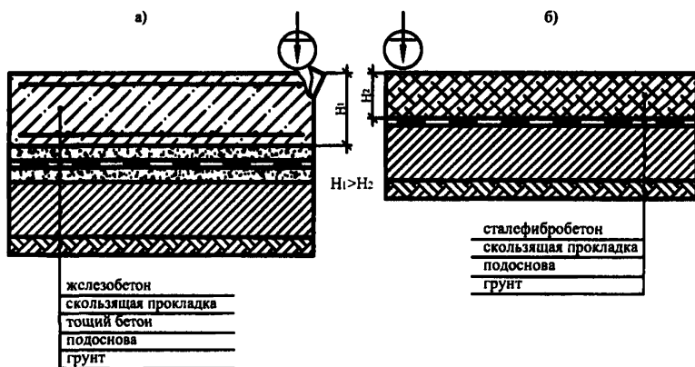
Рис.1. Сопоставительные конструктивные решения промышленных полов по грунтам:
