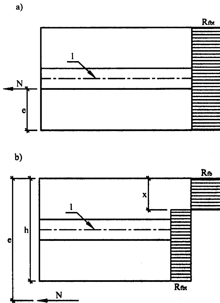
Рис. 7. Эпюры напряжений во внецентренно растянутых элементах прямоугольного сечения а – при приложении продольной силы N в пределах ядра сечения; б – то же, за пределами 1 – стержневая или проволочная арматура
