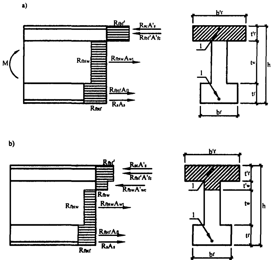
Рис.4. Схема распределения усилий и эпюра напряжений в сечениях, нормальных к продольной оси изгибаемого элемента двутаврового сечения при комбинированном армировании а – при \chi \leq t'_r ; б – при \chi > t'_r
