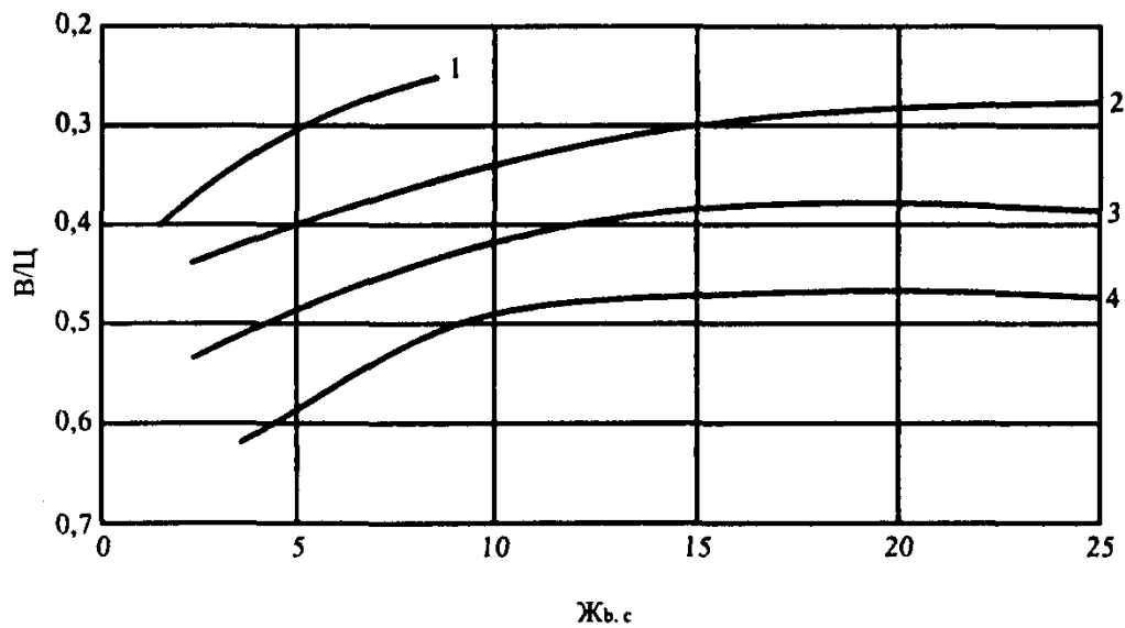
Рис. 1. Графики для подбора отношения Ц:П, обеспечивающего требуемую жесткость сталефибробетонной смеси в зависимости: а – от жесткости исходного бетона при \mu_n : 1-1%; 2-1,5%; 3-2,5%. б – цементно-песчаного отношения Ц:П от жесткости исходного бетона Ж_{б.с} и водоцементного отношения Ц:П равного: 1-1:1; 2-1:2; 3-1:3; 4-1:4.
