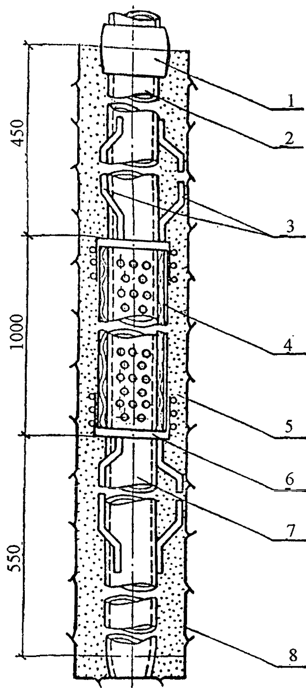
Рис.3. Типовая конструкция водоприемника опусного пьезометра
