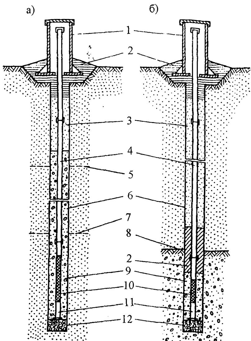
Рис.2. Опускные пьезометры
