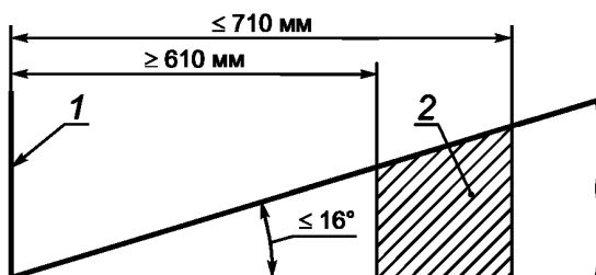
1 — плоскость резания; 2 — допустимая зона расположения переднего светового луча ЭЧПУ
