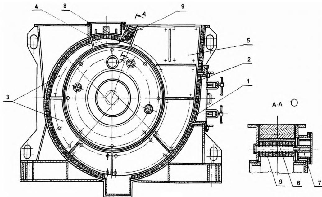
Рисунок 15 – Корпус мельницы MB-1600
