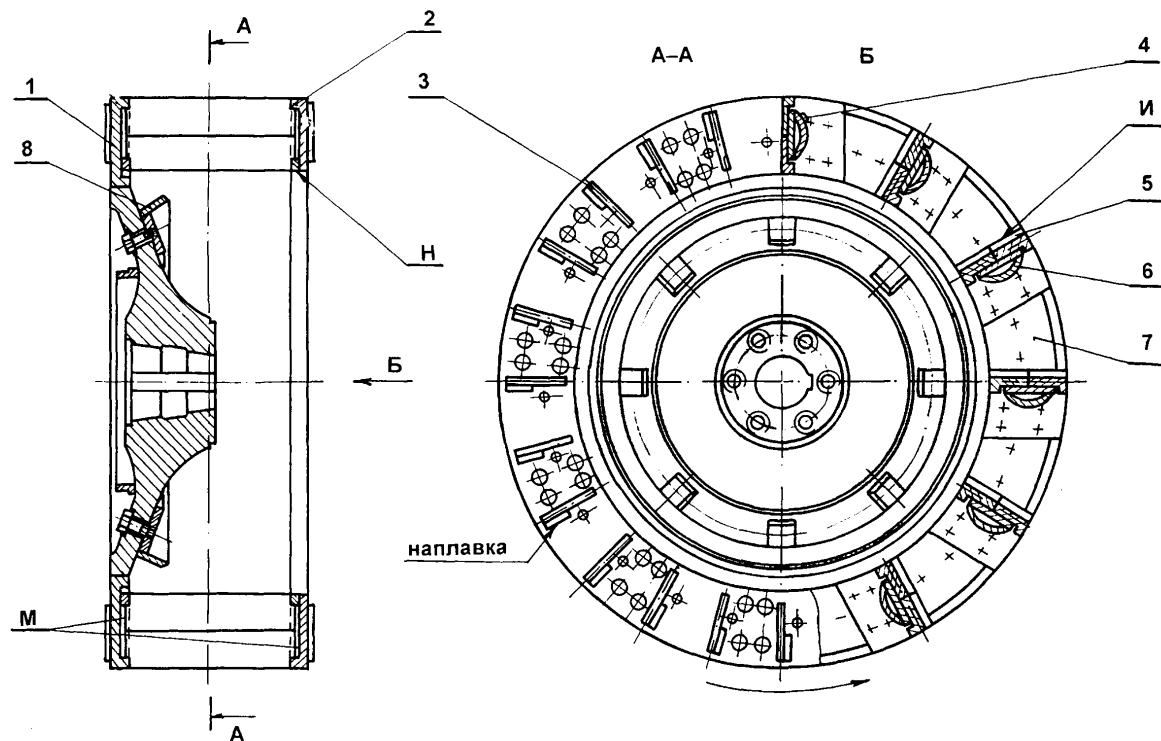
Рисунок 11 – Ротор MB-2120
