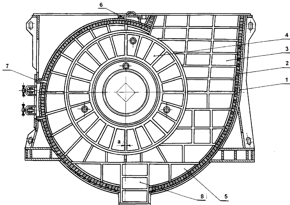
Рисунок 13 – Корпус мельницы MB-3300
