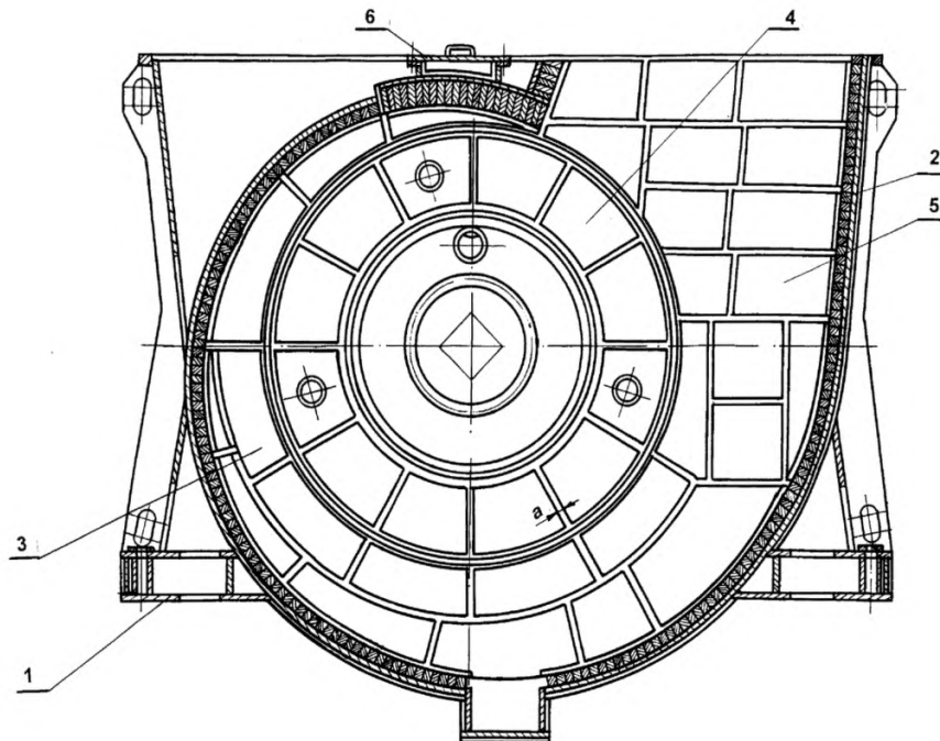
Рисунок 14 – Корпус мельницы MB-2700
