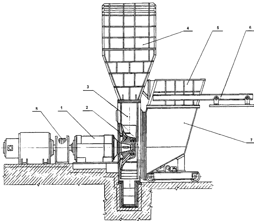
1 – блок подшипников; 2 – ротор; 3 – корпус мельницы; 4 – сепаратор; 5 – патрубок; 6 – шибер отсечной; 7 – патрубок подводящий; 8 – муфта упругая
