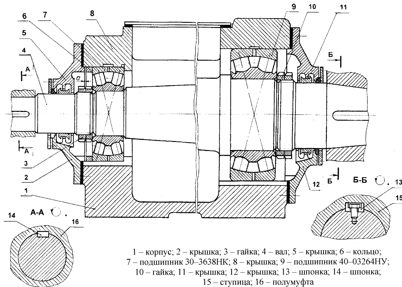
Рисунок 7 – Блок подшипников МВ–2700
