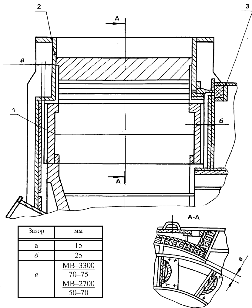
Рисунок 5 – Зазоры между ротором, корпусом и патрубком подводящим
