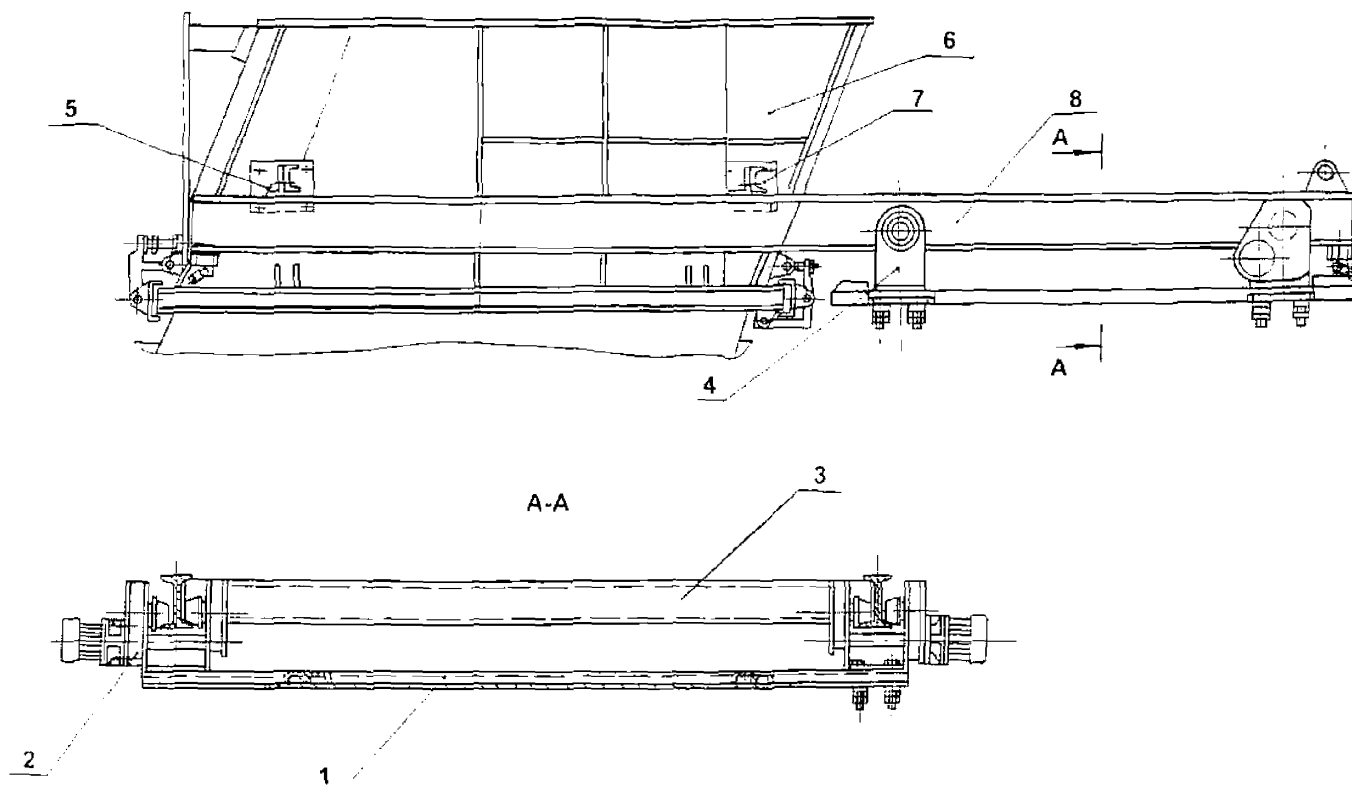
1 – шибер; 2 – тележка приводная; 3 – стяжка; 4 – тележка холостая; 5, 7 – кронштейн; 6 – патрубок; 8 – монорельс
