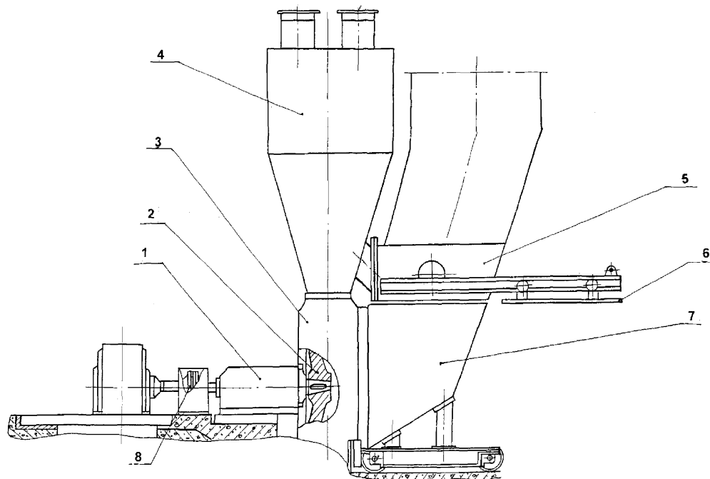
1 – блок подшипников; 2 – ротор; 3 – корпус мельницы; 4 – сепаратор; 5 – патрубок; 6 – шибер отсечной; 7 – патрубок подводящий; 8 – муфта упругая Рисунок 2 – Мельница МВ-2700
