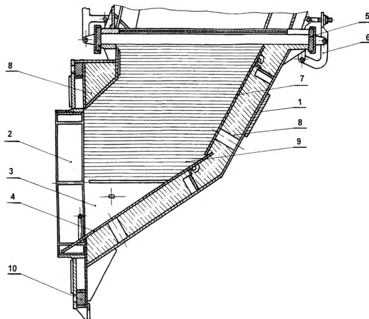
Рисунок 22 – Патрубок подводящий МВ–2120, МВ–1600
