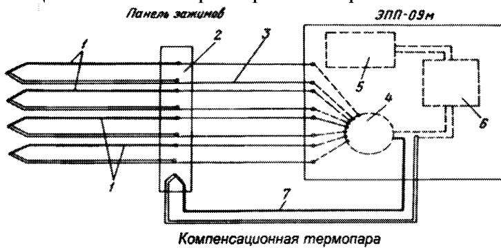
а) схема подсоединения термопар к электронному автоматическому потенциометру
