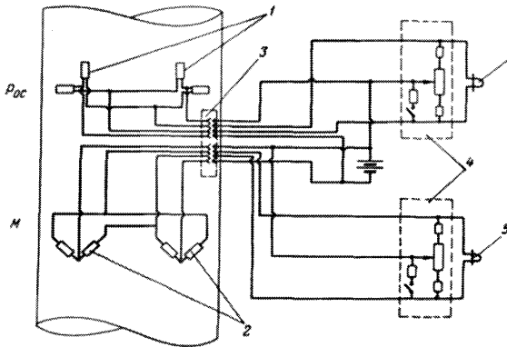
Рисунок Ц.7 – электрическая схема измерений при для определения коэффициента трения
