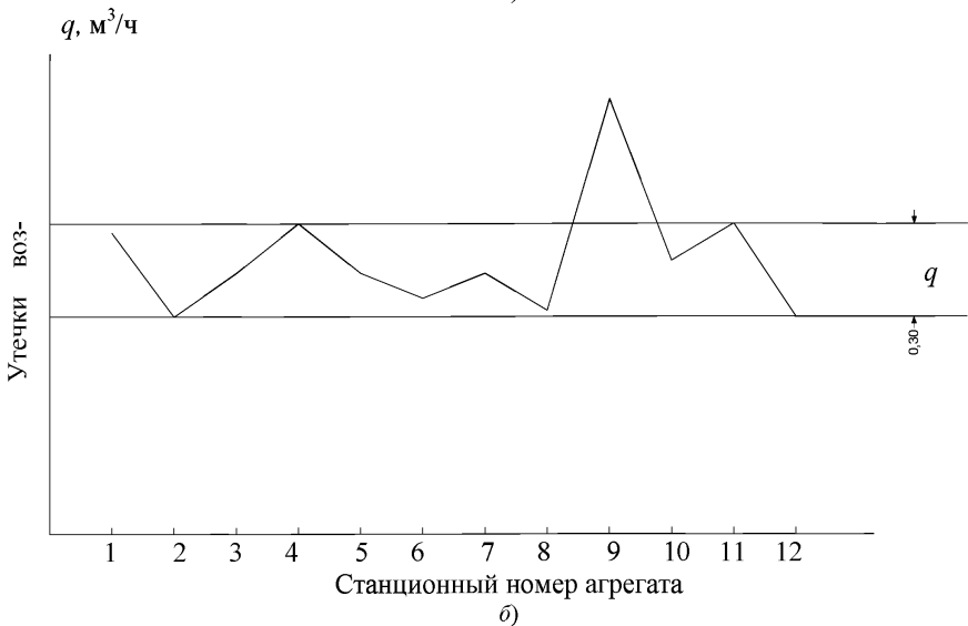
Рисунок Ш.1 – Контроль утечки воздуха из камеры рабочего колеса турбины при работе в режиме СК:
