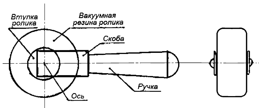
Рисунок Н.2 – Ролик для прикатывания термоэтикеток
