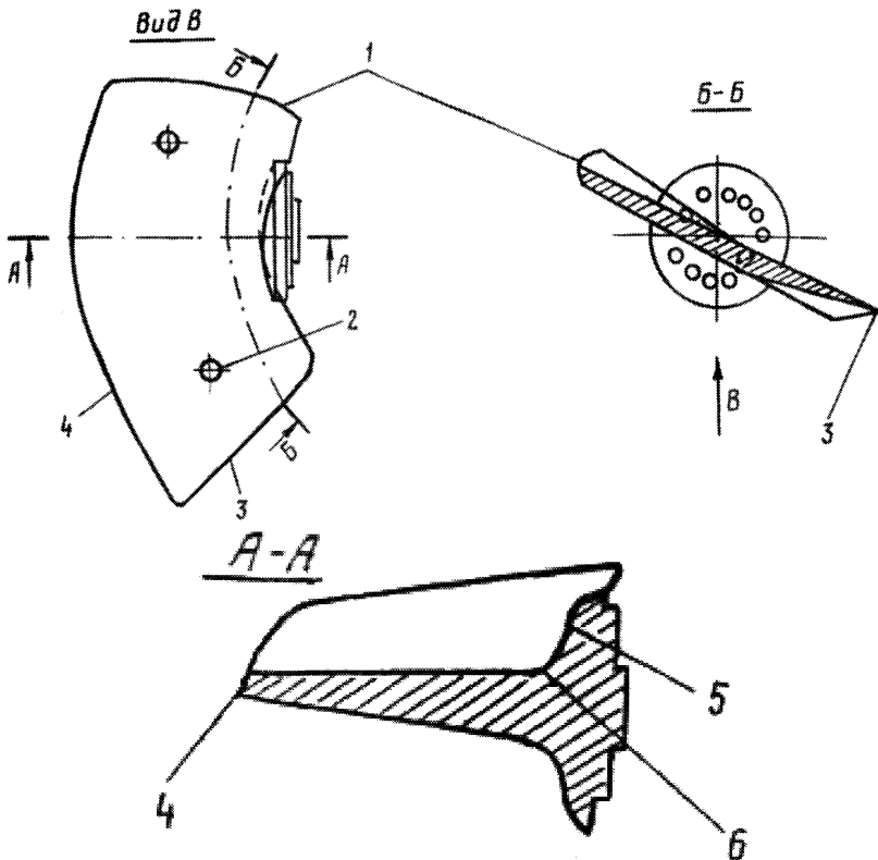
Рисунок ГА.2 – Схема лопасти рабочего колеса поворотно-лопастной гидротурбины с указанием основных мест контроля.
