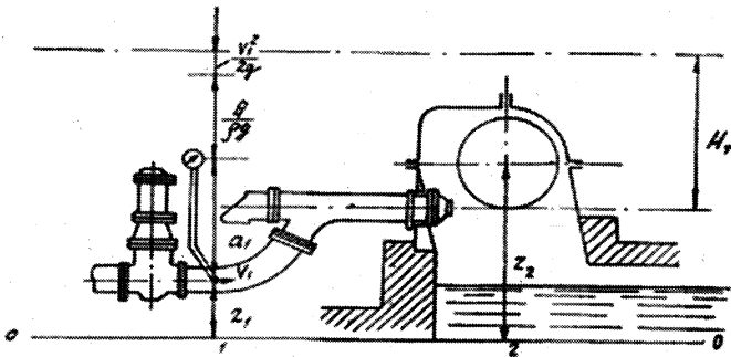
Рисунок А.2 – Схема определения напора
