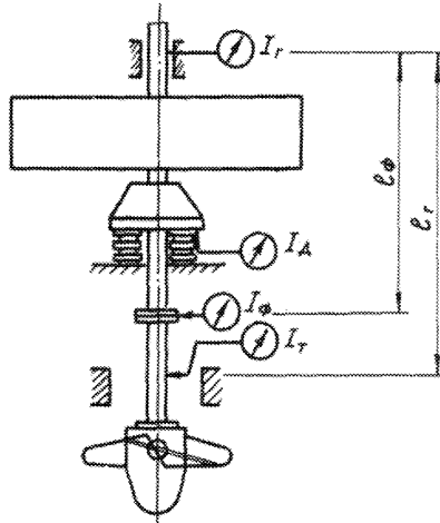
Проверка общей линии валов методом поворота ротора агрегата на 360°
