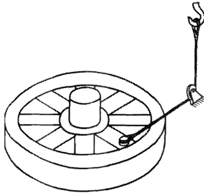
Рисунок Д.2 – Несимметричный способ поворота ротора гидроагрегата
