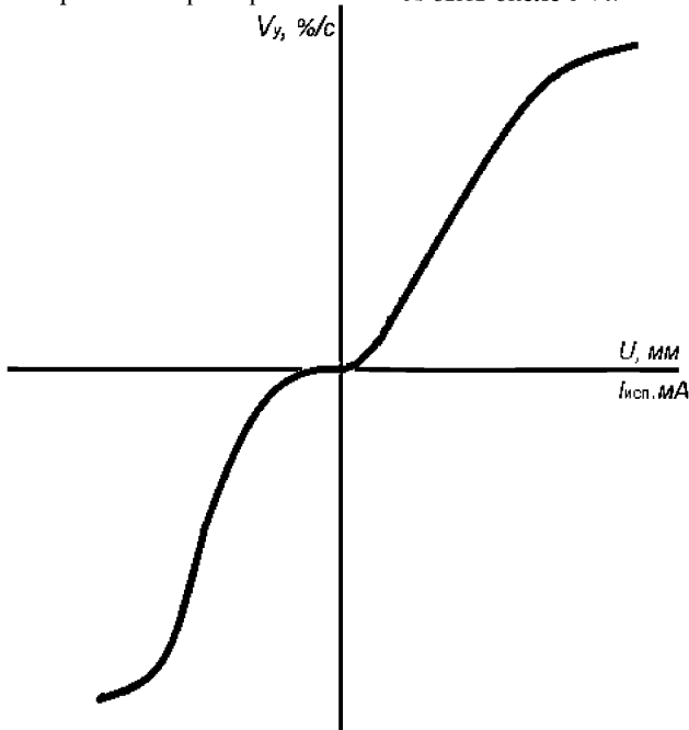
Рисунок Ж.4 – Характеристика главного сервомотора
