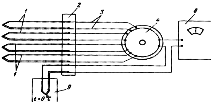
б) схема подсоединения термопар к переносному потенциометру
