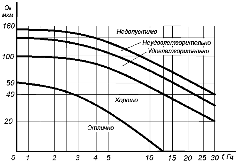
Рисунок И.1 – Оценка вибрации гидроагрегата
