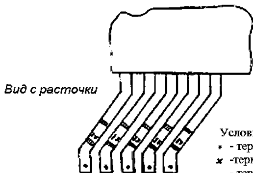
Рисунок Н.3 – Схема установки термопар и термоэтикеток на лобовых частях обмотки статора гидрогенератора.
