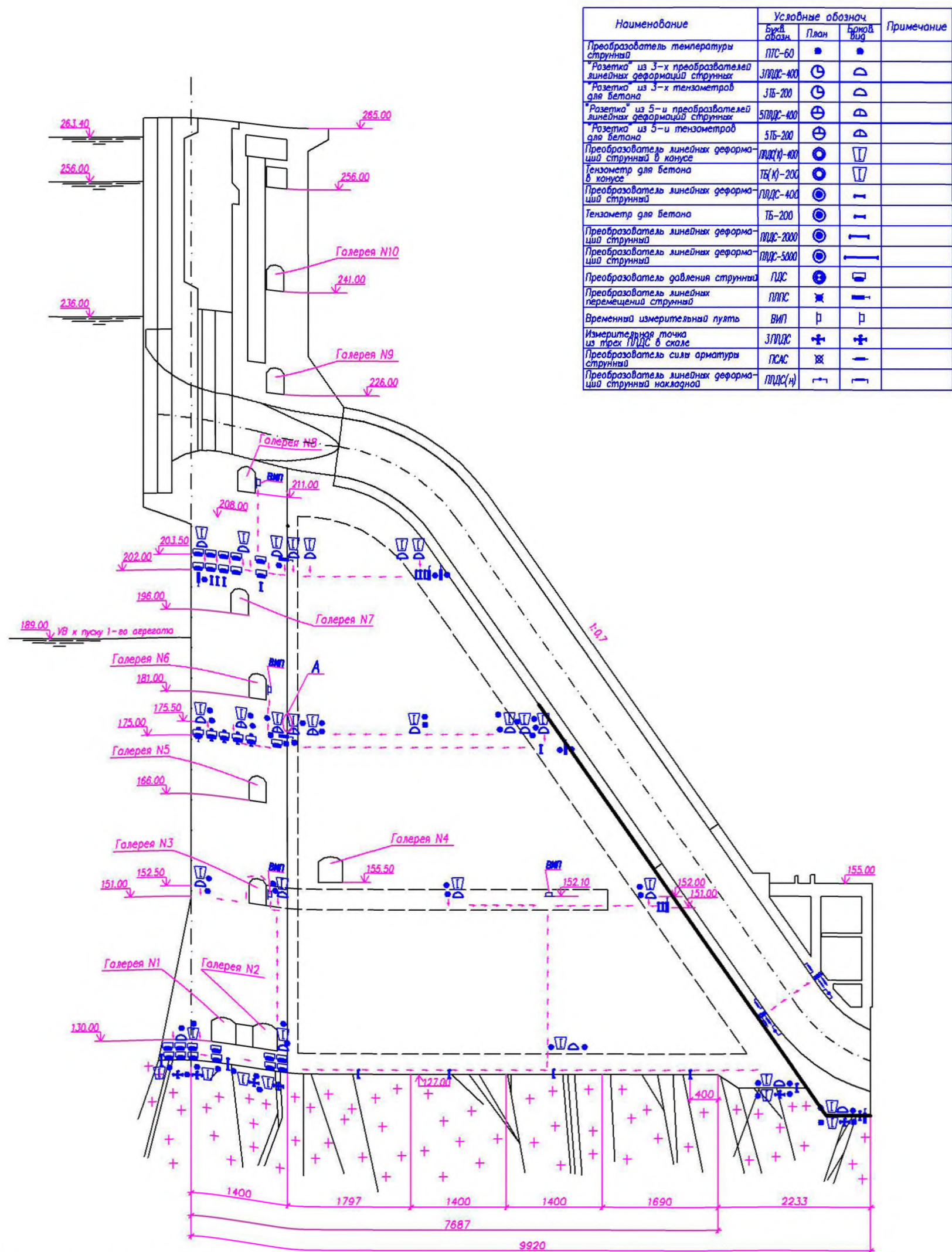
Рисунок. А.1 - Размещение дистанционной КИА в секции бетонной гравитационной плотины
