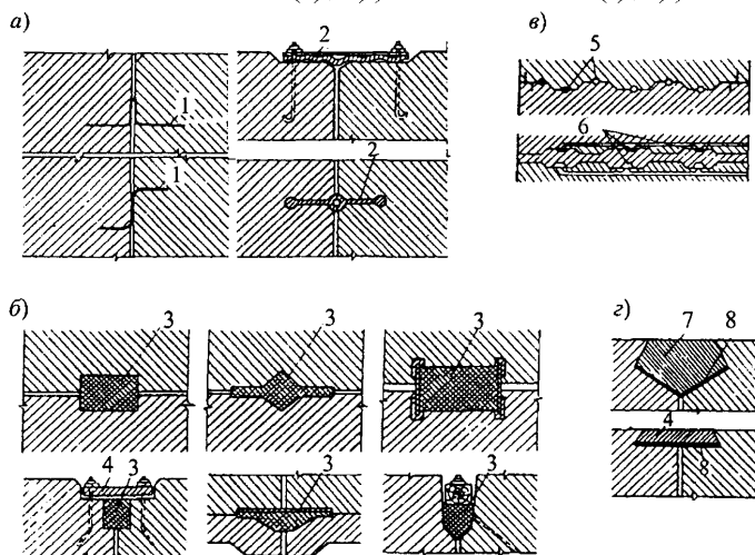
Рисунок К.1 – Схемы расположения уплотнений в постоянных деформационных швах плотин на скальном (а, б) и нескальном (в, г) основаниях
