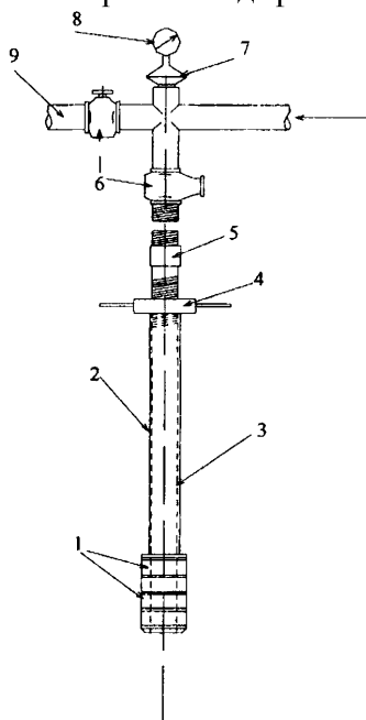
Рисунок Л.3.9 – Площадная инъекция бетона с использованием тампона (при наличии развитой дефектной зоны)
