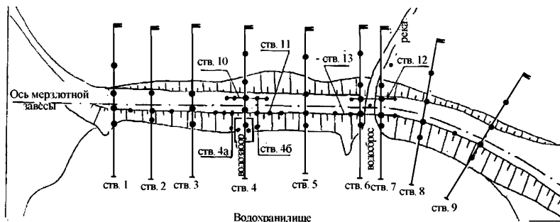
Рисунок Ж.2 – Схема расположения наблюдательных створов температурных скважин на плотине мерзлого типа Анадырской ТЭЦ
