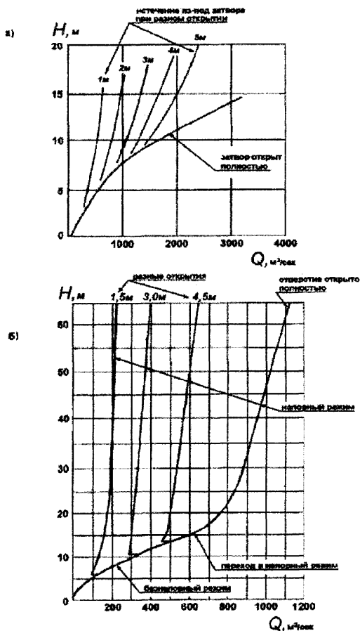
Рисунок И.1 – Характерные формы кривых пропускной способности
