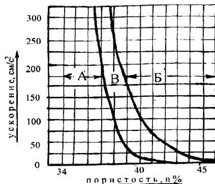
Рисунок Е.9 – Критическое значение ускорения ( a_{кр} , \text{см/с}^2 ) при различной пористости водонасыщенных мелкозернистых песков
