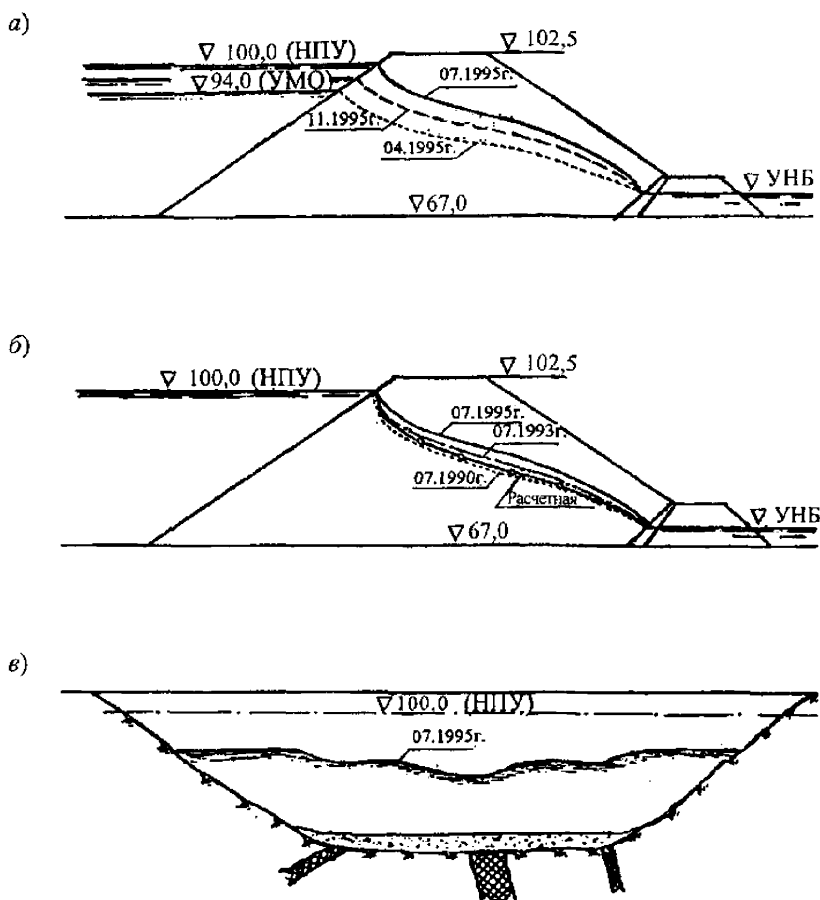
а - в годичном интервале наблюдений; б - в многолетнем интервале наблюдений; в - продольная поверхность депрессии по измерениям в пьезометрических створах Рисунок Д.7 – Кривые депрессии, полученные в результате обработки данных наблюдений
