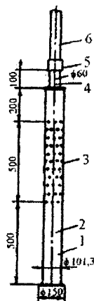
1 – отстойник; 2 – трубка 0-1190; 3 – перфорированная часть, диаметр отверстия 1 мм; 4 – трубка 0-Ц50; 5 – соединительная муфта; 6 – стояк
