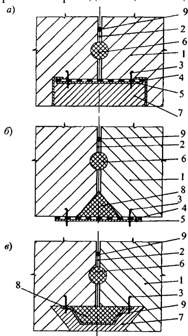
Рисунок К.8 – Ремонт контурных уплотнений
