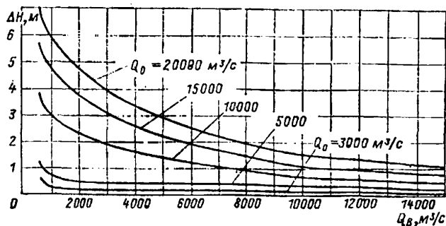
Рисунок И.1.1 – Кривые Q = f(H) в створе Нижегородской ГЭС в зависимости от расхода р. Оки (а) и графики подпора уровня \Delta H при различных расходах Волги Q_B и Оки Q_O (а)
