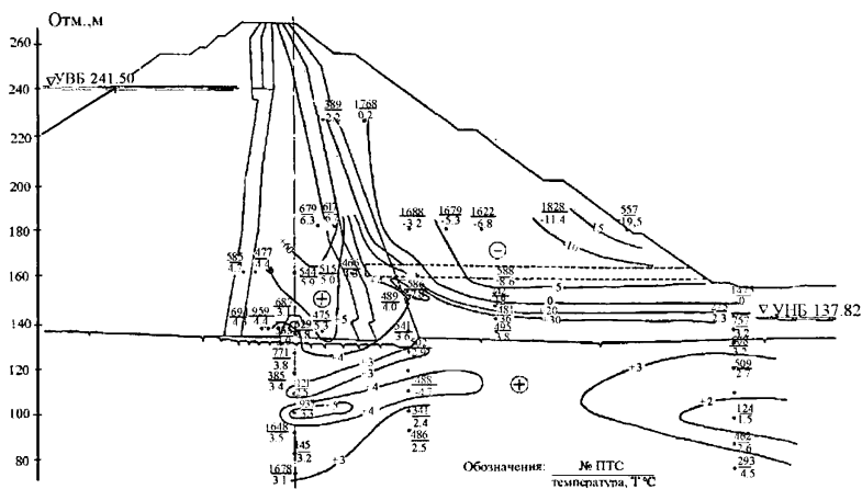
Рисунок Ж.7 – Изотермы в поперечном створе плотины на определенную дату (пример)
