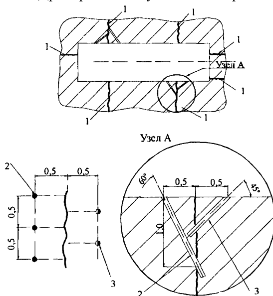
Рисунок Л.3.3 – Дренажное и уплотнение трещин инъекцией
