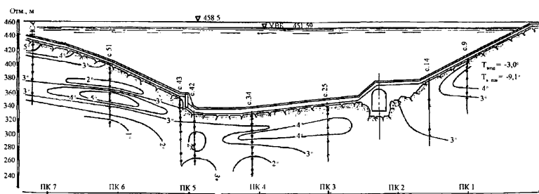
Рисунок Ж.8 – Изотермы в основании плотины на определенную дату (пример)
