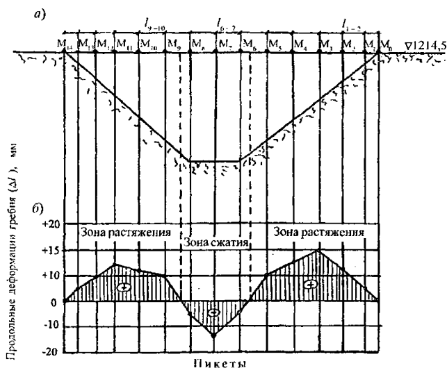
Рисунок Д.5 – Эпюра продольных деформаций гребня плотины
