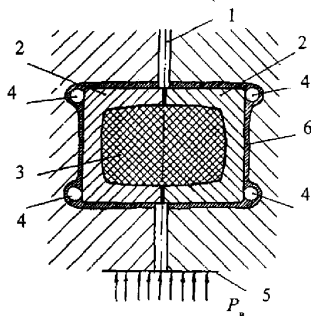
Рисунок К.4 – Восстановление водонепроницаемости уплотнения деформационного шва, выполненного неудаляемыми железобетонными корытами, при наличии обходной фильтрации по контакту железобетонные корыта - бетон сооружения
