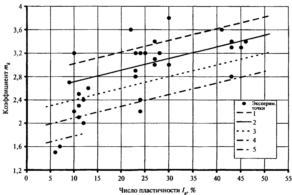
Рисунок 4 — Зависимость коэффициента m_k от числа пластичности I_p и показателя текучести I_L для юрских глинистых грунтов ( n = 32 ; m_k = 2,51 + 0,02I_p - 1,24I_L ; R = 0,83 ; S = 0,38 ): I_L : 1 — (-0,25) ; 2 — 0,0 ; 3 — 0,25 ; 4 — 0,5 ; 5 — 0,75
