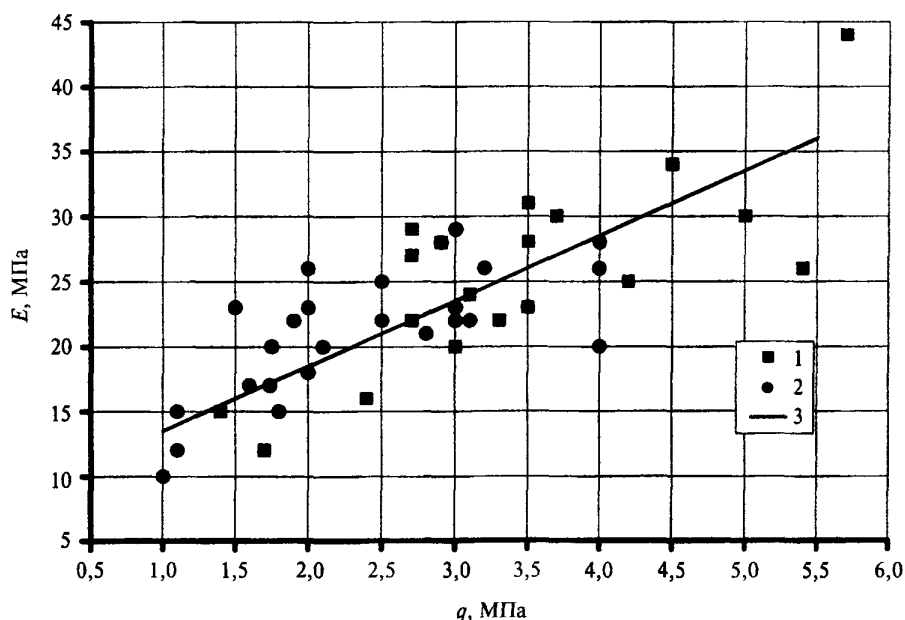
Рисунок 2 — Зависимость модуля деформации E по данным штамповых и прессиометрических испытаний от удельного сопротивления грунта под конусом зонда q для юрских глинистых грунтов:
