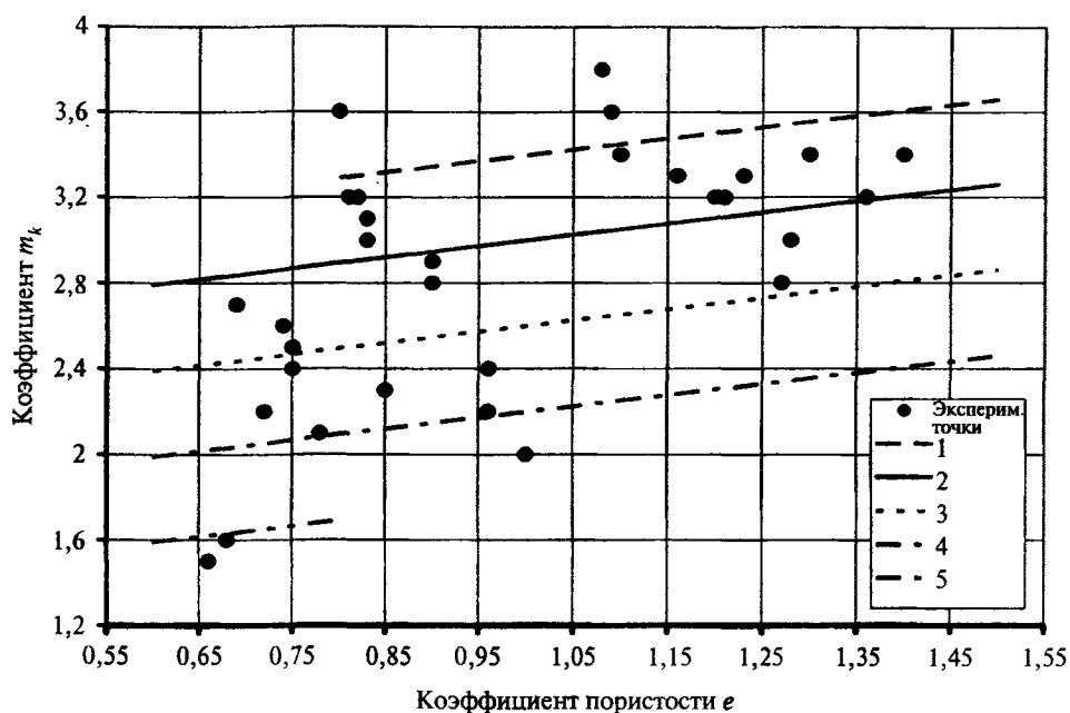
Рисунок 3 — Зависимость коэффициента m_k от коэффициента пористости e и показателя текучести I_L для юрских глинистых грунтов ( n = 32 ; m_k = 2,47 + 0,53e - 1,60I_L ; R = 0,79 ; S = 0,42 ): I_L : 1 — (-0,25) ; 2 — 0,0 ; 3 — 0,25 ; 4 — 0,5 ; 5 — 0,75
