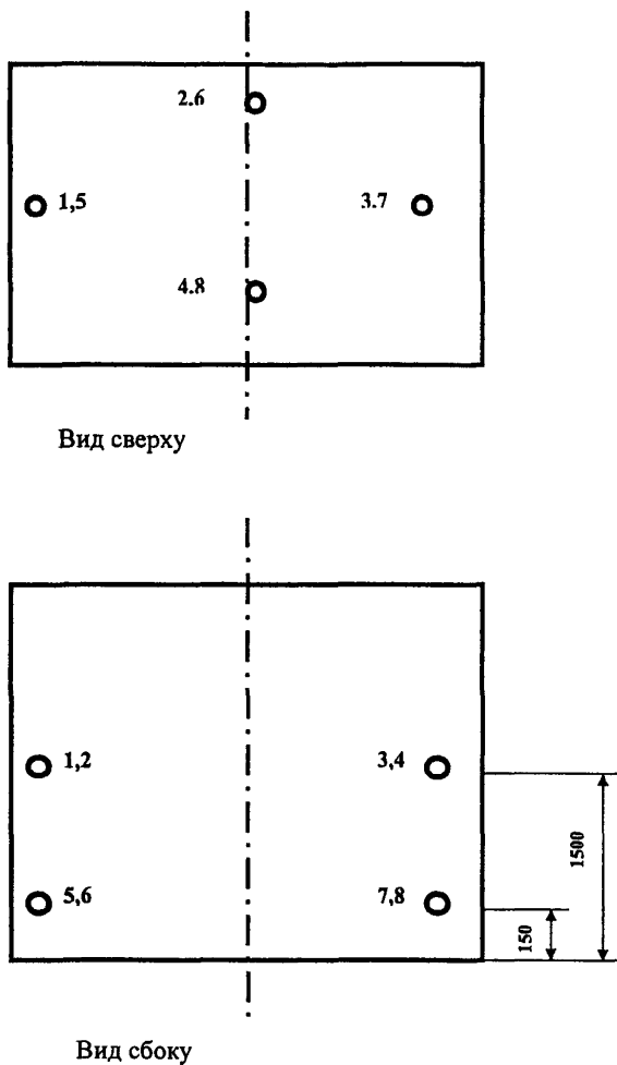
Рис. 1. Места установки датчиков температуры воздуха в помещениях площадью до 12 м 2 .
