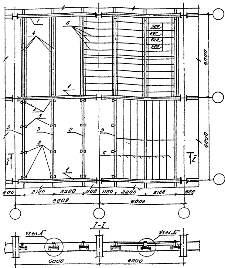
Рис.8. Монтажная схема металлических балок перекрытия и план опалубки. Вариант по металлическим балкам перекрытия.
