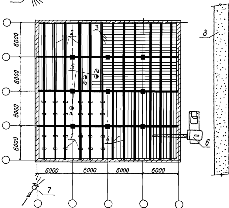
Рис.1. Схема организации работ
