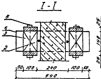
Рис.4. Подвесная опора и тяга. Вариант по сборным железобетонным балкам перекрытия.
