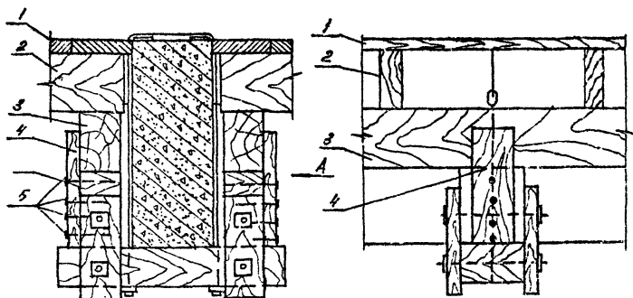
Рис. 5. Узел "Б" Вариант по сборным железобетонным балкам перекрытия.
