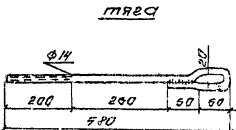
Рис.4. Подвесная опора и тяга. Вариант по сборным железобетонным балкам перекрытия.
