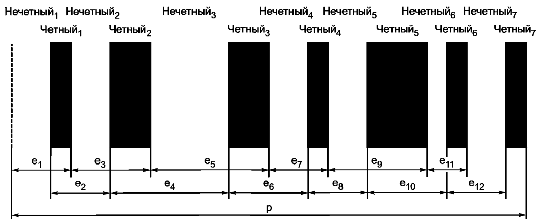
Рисунок 9 — Измеряемые параметры при декодировании
