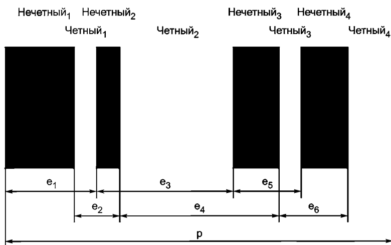
Рисунок 14 — Измеряемые параметры ширины при декодировании
