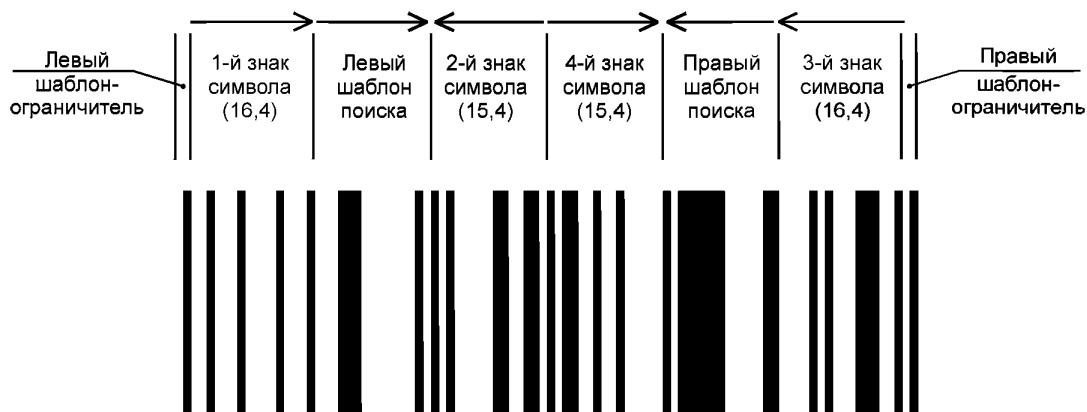
Рисунок 2 — Линейный символ GS1 DataBar Всенаправленный, представляющий номер (01)04412345678909
