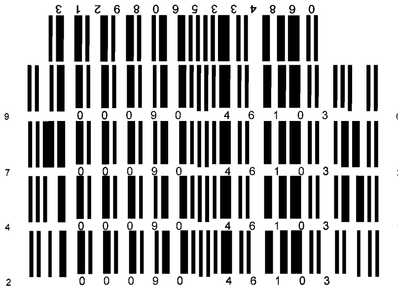
Рисунок Н.2 — Прецеденты для символов URC-A (с префиксами 09, 07, 04 и 02), которые могут быть источником проблем
