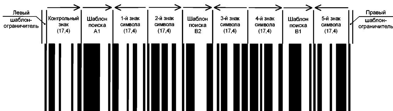
Рисунок 11 — Символ GS1 DataBar Расширенный, представляющий номер (01)90012345678908(3103)001750
