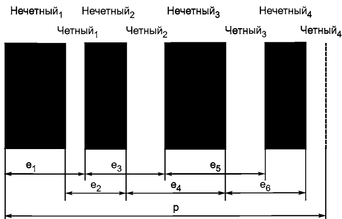
Рисунок 3 — Измеряемые размеры при декодировании
