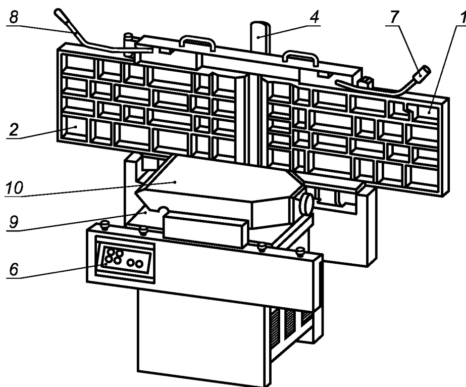
Рисунок 1b) — Пример использования фуговально-рейсмусового станка при рейсмусовании
