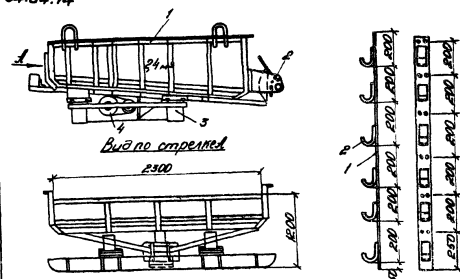
Рис. 4 Вибропитатель: 1-бункер; 2-секторный вибратор; 3-нижняя рама; 4-маятниковый вибратор
