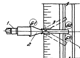
Рис. 9 Схема размещения в рабочей зоне вибратора, виброжелоба, автосамовала и обочины живущего персонала вибраторов, расположенных перпендикулярно ленточному фундаменту
