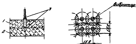
Рис. 7 Уплотнение бетонной смеси внутренним вибратором Рис. 8 Схема престановки вибратора 1-уплотняемый слой; 2-ранее уплотненный слой; 3-предельное положение вибратора R-радиус действия вибратора
