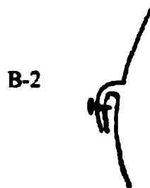
В-2 Края загнуть после монтажа для предотвращения затека-ния влаги и отторачивании винтов
