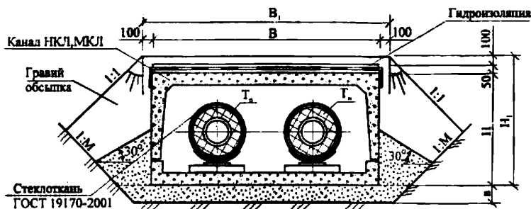
Тп - подающий трубопровод отопления; Т0 - обратный трубопровод отопления;
