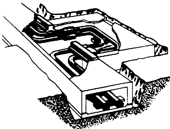
Рисунок 5 - Гнутые компенсаторы
