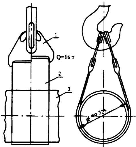
1 - пластина; 2 - лента; 3 – трубопровод Рисунок 3 - Полотенце мягкое
