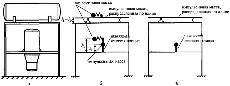
Рисунок 9.1. Постамент с двумя сосудами и соответствующие расчетные схемы
