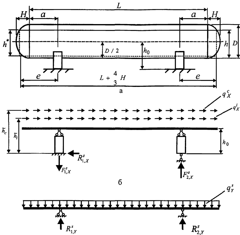
Рисунок 8.2. Расчетная схема для определения нагрузок на седловые опоры и усилий в обечайке горизонтального сосуда
